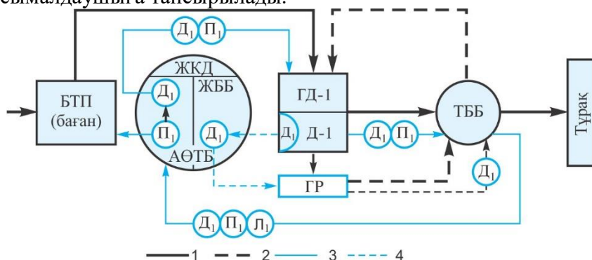
38.1-сурет Диагностикалаумен ТҚК-1 технологиялық процесінің ақпараттық қамтамасыз еу сұлбасы:
