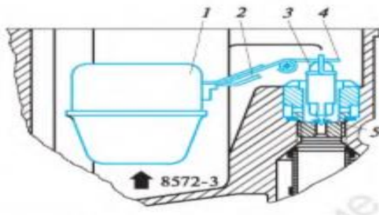
16.3. сурет К-151 карбюраторының өзгермелі механизміні реттеу:
