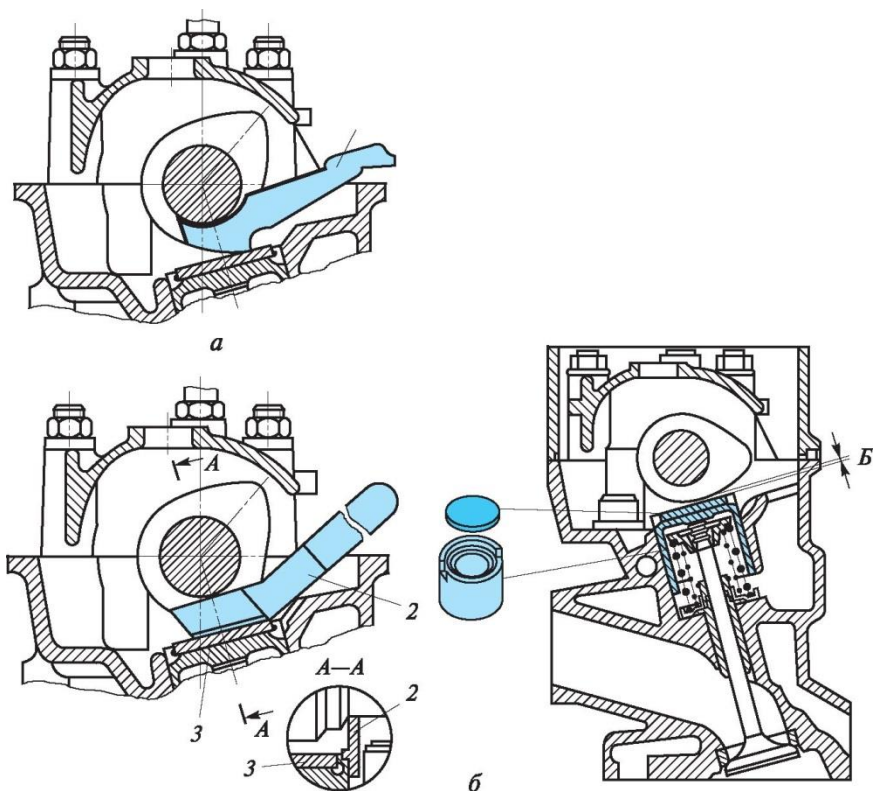
14.7 сурет. ВАЗ-2108, -2109 қозғалтқышының тарату механизмінде саңылауды реттеу: а — жақтауды орнату; б — саңылауды бақылау; 1 — жақтау; 2 — фиксатор; 3 — реттеуші шайба; Б — саңылау
