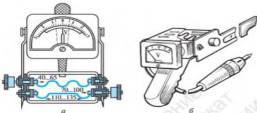
18.2. сурет. Жүктеме ашасы (а) және Э-107 аккумуляторлық сынамасы (б)
