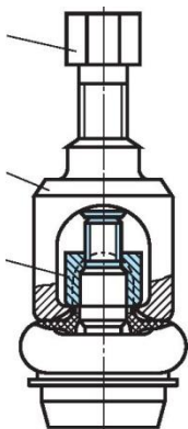
21.8 сурет. Рульдік роликтің ұшын шар желегінен шығаратын алынғыш: 1 — бұрылу рычагы; 2 — корпус; 3 — бұрама
