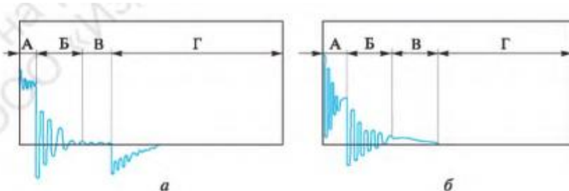
18.5. сурет. Тұтану жүйесі шынжырларының осциллограммасы: а – алғашқы; б – екінші.
