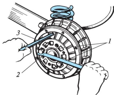
21.12 сурет. Артқы тежегіштегі тежегіш тежегіштің тежегіш барабанының айтарлықтай тозуымен (коллектордың қалыптасуы):
