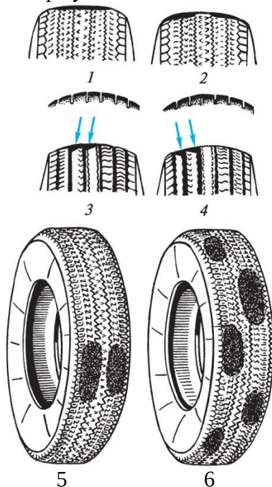
20.17 сурет. Шиналардың табиғи емес тозуының түрлері:
