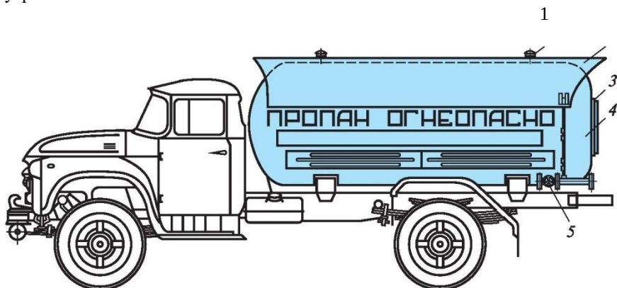
24.2 сурет. Сұйытылған газдарды тасымалдау үшін автомобильді цистерна СГТАЦ-6:
