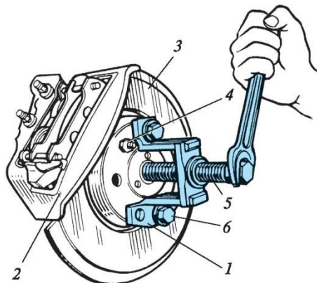
1 — құралдың тұтқасы; 2 — тежегіш тұтқасы; 3 — тежегіш дискі; 4 — сүккыш; 5 — бұрама; 6 — бұрандама
