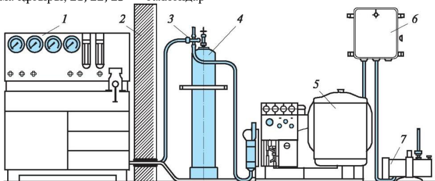
24.6 сурет. Автомобильдердің газдық жабдыкталуын тексеру станді: 1 — аспаптық таған; 2 — шымылдық; 3 — айкастырма; 4 — ресивер; 5 — КР-2 электрокомпрессоры; 6 — жабдыкталу шкафы; 7 — 2НВР-5Д вакуумдық сорап
