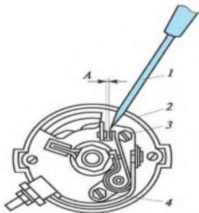
18.3. сурет. байланыстарды үлестіруші арасындағы саңылауларды реттеу: 1 – бұрауыш, 2 – үлестіруші, 3,4 – бұрандалар, А – байланыстар арасындағы саңлақ
