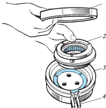
19.24 сурет. Синхронизаторды сұққыларды радиусты шегелеуге арналған арнайы жабдыққа орнату:
