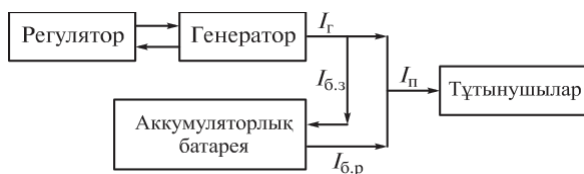
3.2 сур. Электр жабдықтау жүйесінің құрылымдық сызбасы:
