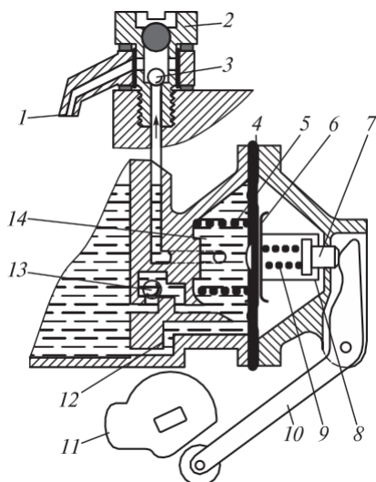
2.47 сур. Диафрагмалық тездеткіш сорғысы бар карбюратор:
