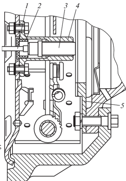
484 сур. Дөңгелектің бұрыштық айналу жылдамдығының бергіші: 1 — жетек; 2 — тығыздағыш; 3 — электромагниттік бергіш; 4 — тіреуіш; 5 — ротор (бергіш коздырғышы)
