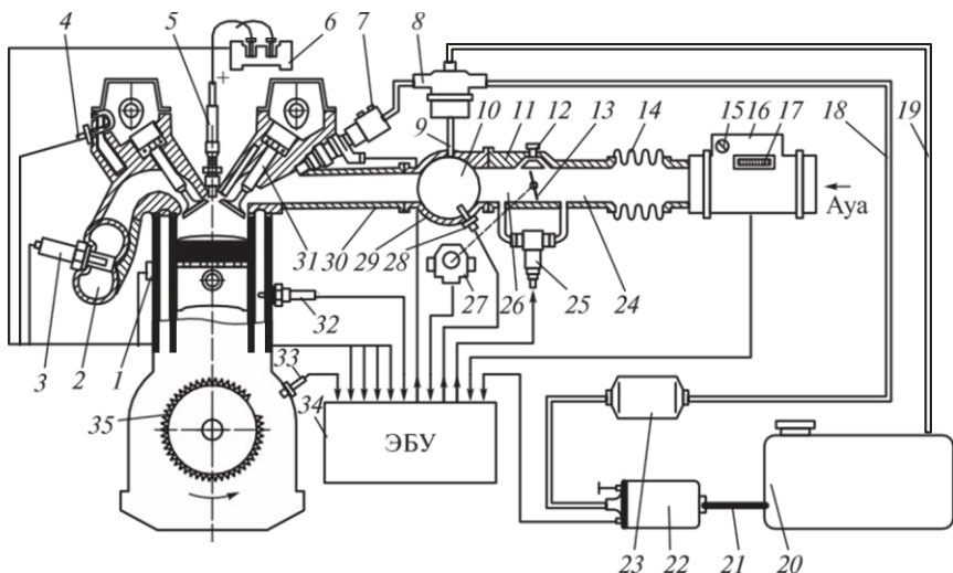
2.58 сур. ЗМЗ-4062.10 қозғалтқышындағы отынды тікелей бүрку жүйесінің жалпы сызбасы:
