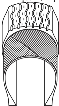
4.131 -сурет. Диагональді шина
