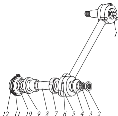
4.54 сур. Реактивті қарнақ: 1 — май құйғыш; 2 — сомын; 3 — серіппелі тығырық; 4 — тығыздама; 5 — қарнақ; 6 — тойтарма шеге; 7, 9 — ішкі және сыртқы ішпектер; 8 — сұкқы; 10 — серіппе; 11 — төсем; 12 — қақпақ
