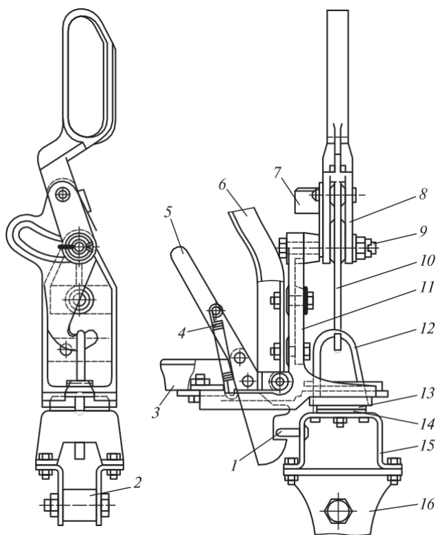
4.119 -сурет. Кабинаның ілмекті құрылғысы:
