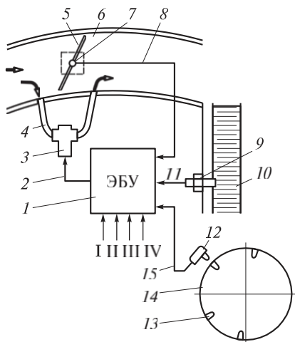
264 сур. Бос жүріс жүйесінің сызбасы: 1 — электронды басқару блогы (ЭББ); 2 — ЭББ бос жүріс реттегішіне келетін дабыл (электромагниттік клапан); 3 — бос жүріс реттегіші; 4 — бос жүрісте жұмыс істейтін айналма арнасы; 5 — кедергі қалқаны; 6 — кіріс коллекторы; 7 — кедергі қалқаны тәртібінің бергіші; 8 — кедергі қалқаны тәртібі туралы ЭББ ға дабыл; 9 — салқындату сұйықтығы температурасының бергіші; 10 — сақyndатылу жидесі; 11 — салқындату сұйықтығы температурасын туралы ЭББға келетін дабыл; 12, 13 — иінді білік айналуы; 14 — иінді білік; 15 — иінді білік айналу жиілігі туралы ЭББға келетін дабыл; I — IV — басқару блогына келетін кіріс дабылдары; ■ = > — ауа қозғалысы
