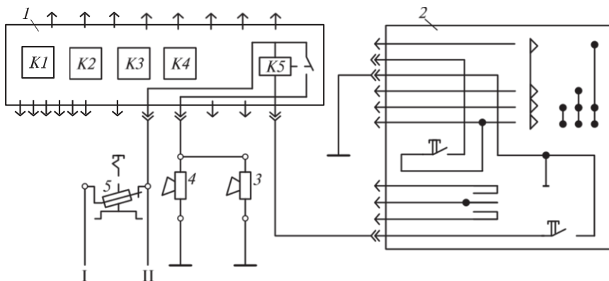
3.32 сур. КамАЗ автомобилінің үндестік дыбыстық сигнализациясын қосу сызбасы:
