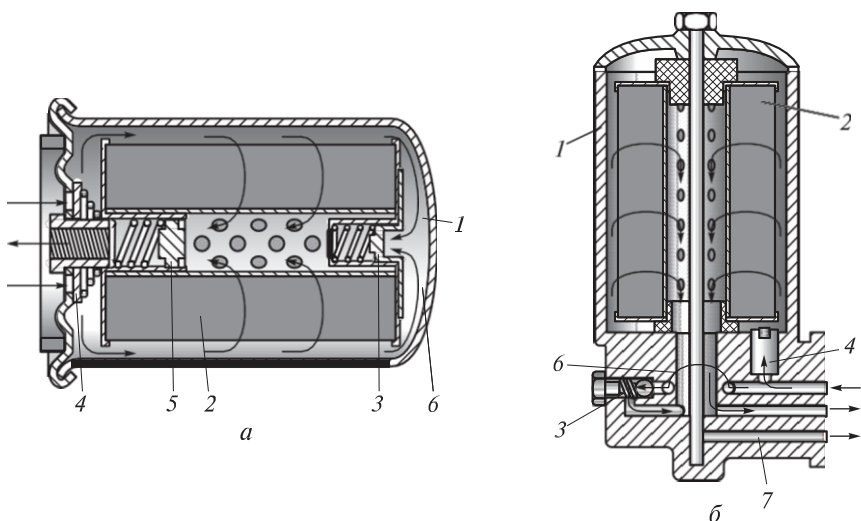
2.34 сур. Бөлшектенбейтін (а) және бөлшектенетін (б) толық ағынды көлемді-сорылатын сүзгілер:
