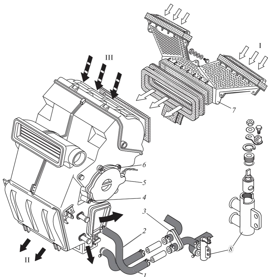
4.122 -сурет. Құбырлы жылытқыш:
