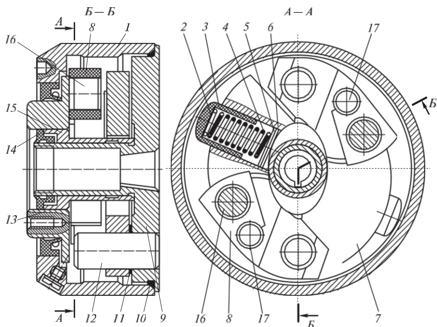
2.81 сур. Отынды бүркуін алдын алуының автоматты түрдегі жалғастырғыштың құрылғысы:
