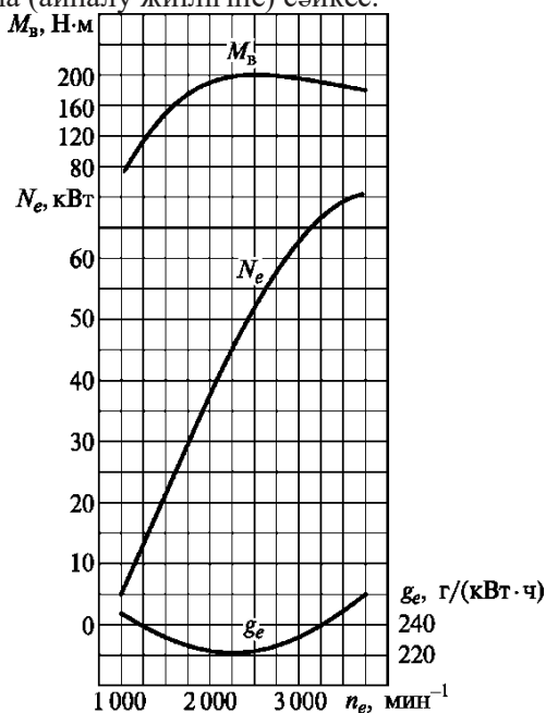
25. сур. ГАЗ-560 төртцилиндрлік қатарлы дизельдің сыртқы сипаттамасы:
