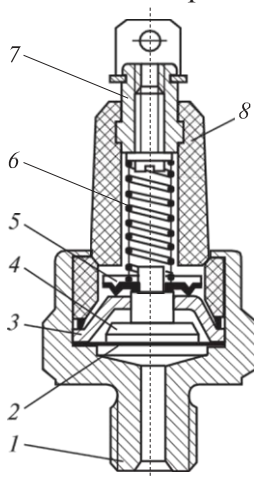
4.100 -сурет. Қысымды апаттық төмендету бергіші:
