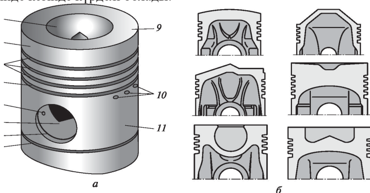
29 .сур.Дизель піспекі (а) жәнәтүрлі қозғалтқыштар піспектерінің пішіндері (б): 1 — төменгі май алғыш сақинаның жырашығы; 2 — тоқтату сақинасына арналған бұнақ; 3 — дөңсешенің ішкі беті; 4 — піспектік сақинаны майлау үшін саңылау; 5— жоғары май алғыш сақинаның жырашығы; 6 — сығымдауыш сақиналардың жырашықтары; 7 — піспектің бастиегі; 8 — піспектегі жану камерасы; 9 — піспектің табандығы; 10 — майды бұруға арналған саңылау; 11 — етек
