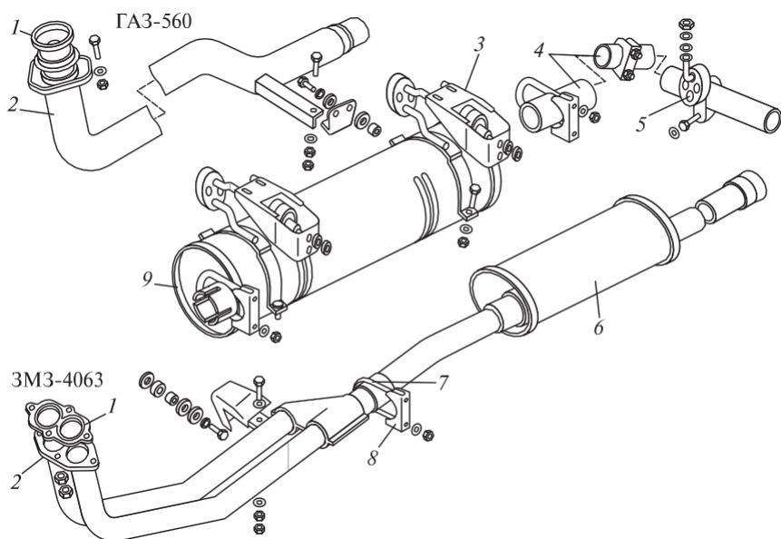
2.94 сур. ГАЗ-3302 жүк автомобилінің («Газель») пайдаланылған газды шығару жүйесінің жалпы сызбасы:
