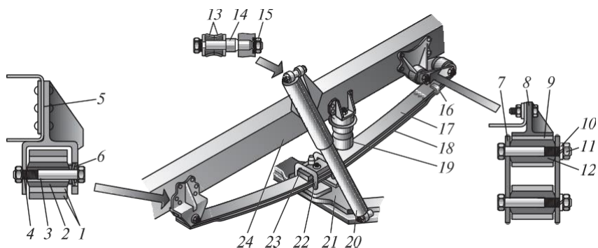
4.44. сурет. ГАЗ-3302 автомобилінің алдыңғы табақты рессоры:
