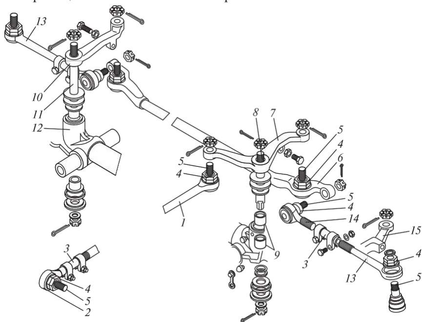
4.59. сурет. ГАЗ-2752 «Соболь» автомобилінің меңгерік жетегі:
