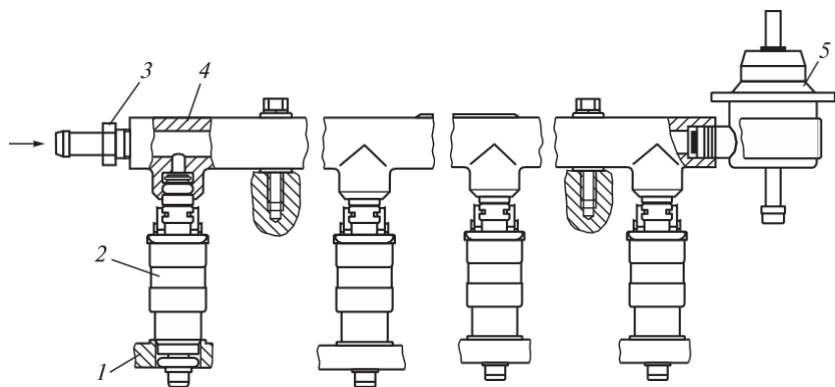
2.63 сур. Кіріс құбыр желісі (коллектор) мен отын құбыр желісі арасындағы бүріккіштердің қондырғысы:
