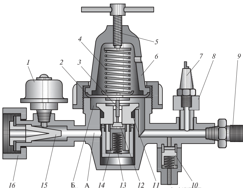
2.55 сур. Жоғары қысымды газ бәсеңдеткіші ЖҚГБ
