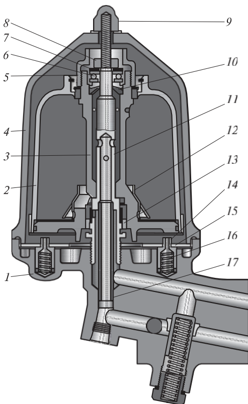
2.35 сур. Ортақ тепкіш сүзгі:
