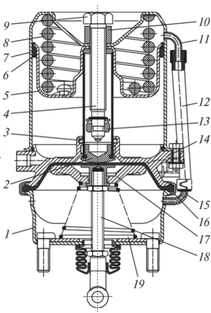
4.90 -сурет. Пневмосеріппелі қуат беру аккумуляторы бар тежегіш камера:
