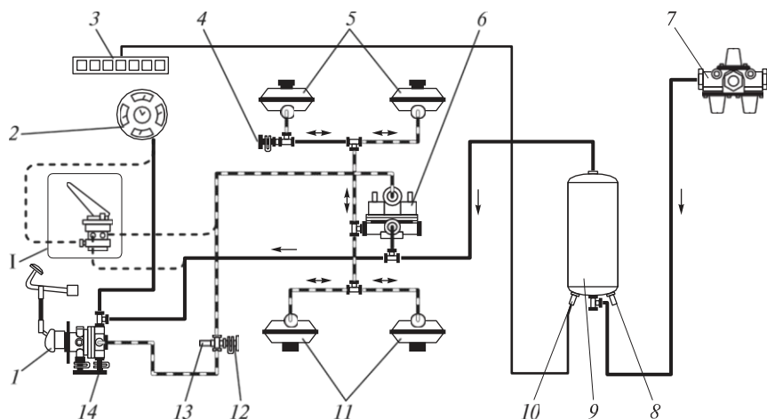
4.107 -сурет. Алдыңғы осьтің жұмыс тежеуіштері жетегі контурының сызбасы: 1 — екі секциялы тежегіш кран; 2 — құрамдастырылған аспап; 3 — бақылау шамдарының блогы; 4, 12, 14 — шығысты бақылау клапандары; 5, 11 — тежеуіш камералары; 6 — тездеткіш клапан; 7 — үш қорғағышты клапан; 8 — конденсатты ағызу клапаны; 9 — ауа жинаушы баллон; 10 — қысымды төмендеті датчигі; 13 — қысым датчигі; А — екі секциялы тежегіш кранның нұсқасы; —►— ауа қозғалысы
