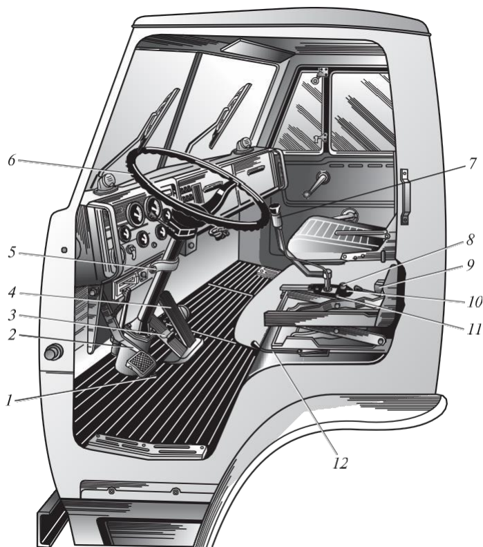
4.116 -сурет. КамАЗ автомобилінің кабинасы:
