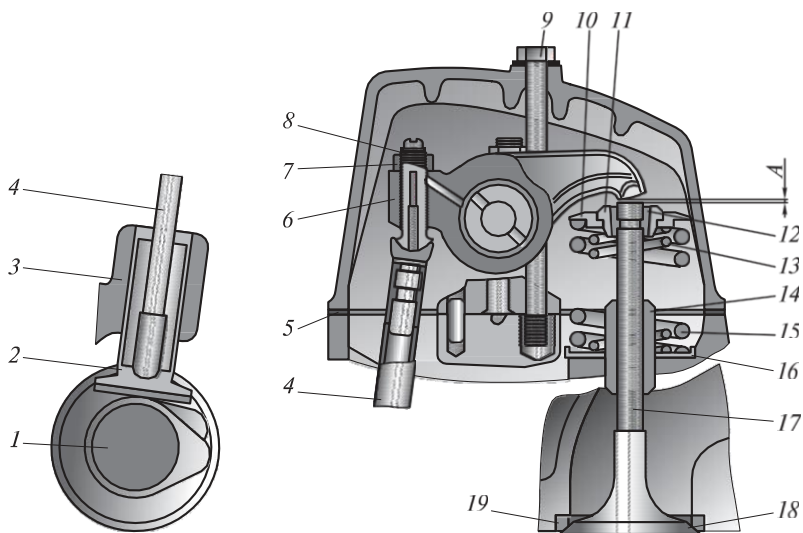
2.18 сур. Газ тарату механизмі:
