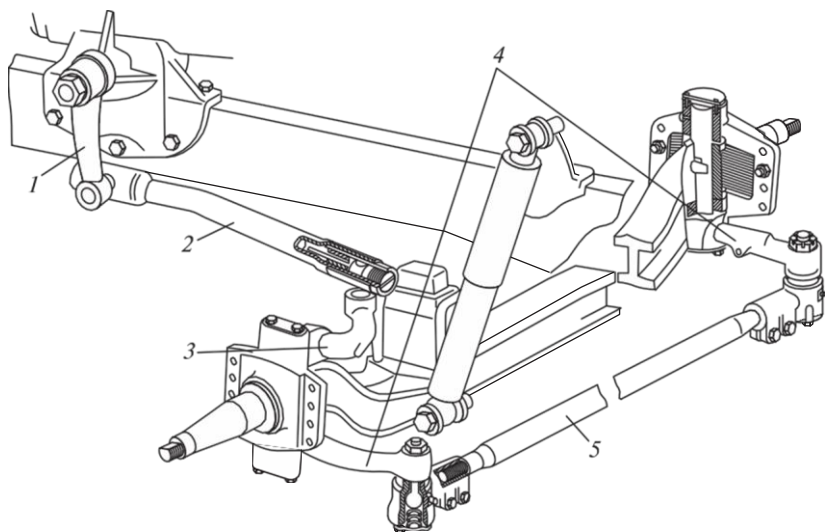
4.67. сурет. ЗИЛ-5301 автомобилінің меңгерік жетегі:
