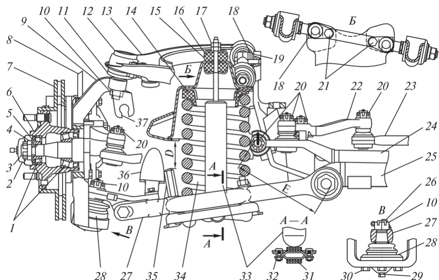
4.40. Алдыңғы аспа:
