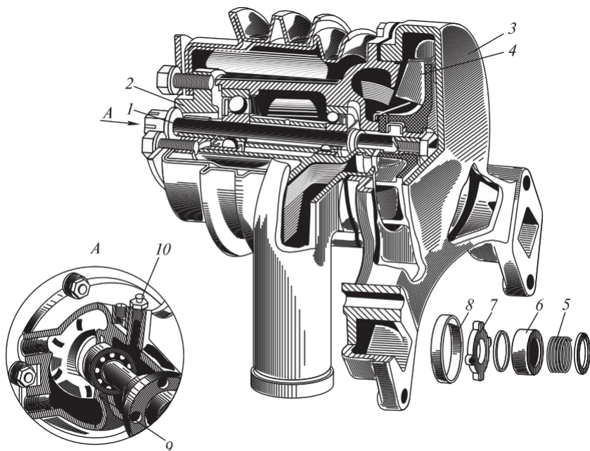
2.29 сур. Ортақ тепкіш түрлі су сорғышы:
