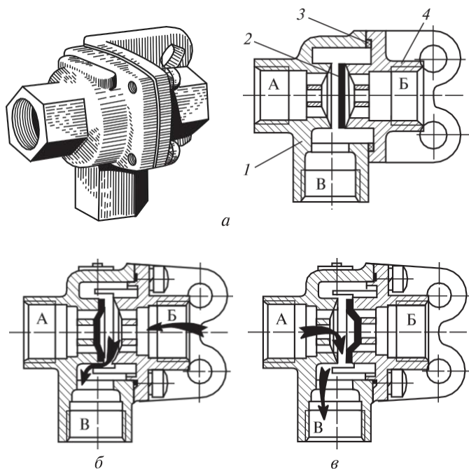
4.109 -сурет. Екімагистральді клапан: а — бастапқы күй; б — тездеткіш клапаннан ауаны жеткізу; в — авариялық тежеу шүмегінен ауаны жеткізу; 1 — корпус; 2 — клапан; 3 — клапанның тығыздағыш сақинасы; 4 — қақпақ; А, Б, В — шығыстар
