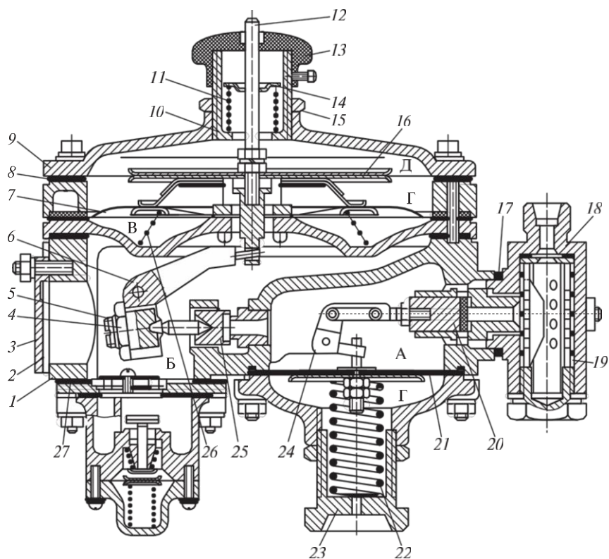
2.56 сур. Төмен қысымды газ бәсеңдеткіші (ТҚГБ):
