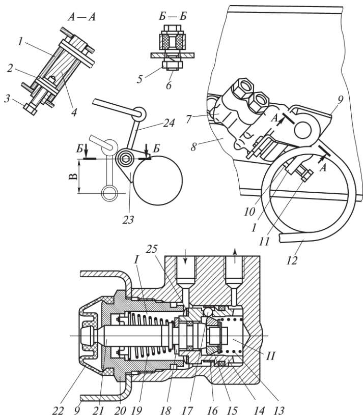
4.77 -сурет. Тежегіш күшін реттегіш автомобиля ГАЗ-3302 «Газель» автомобилі тежеуіш күштерінің реттегіші:
