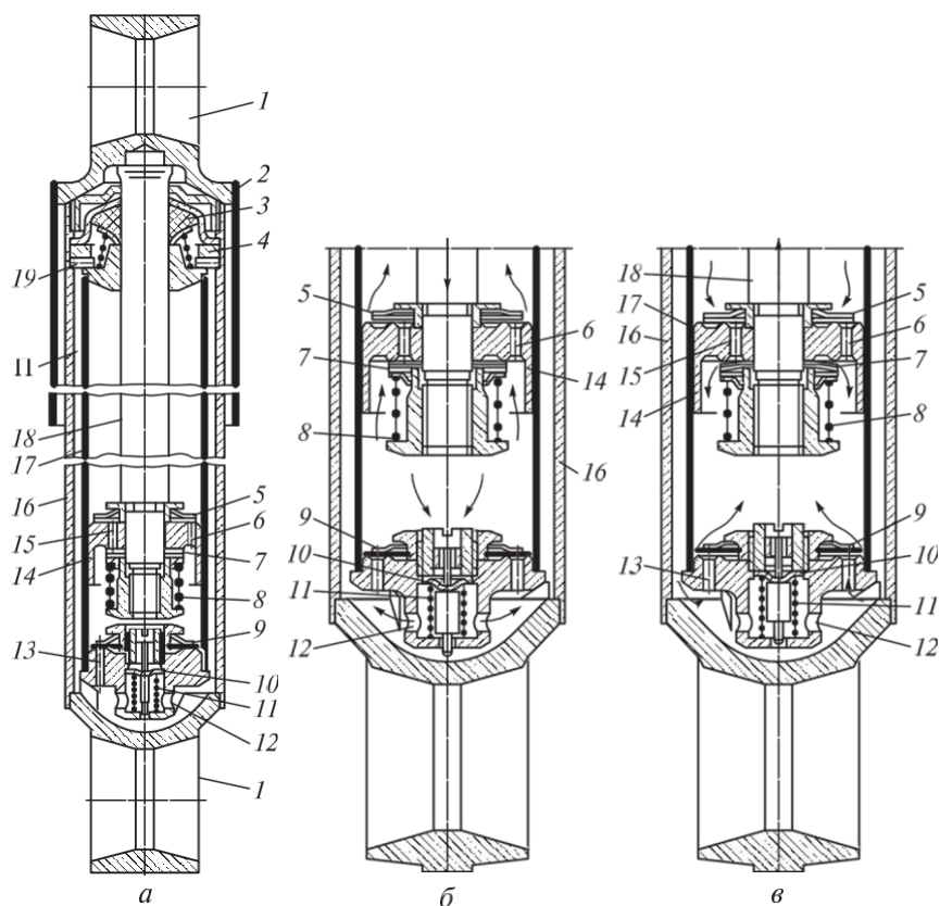
4.49. КамАЗ автомобильдерінің телескоптық косқұбырлы амортизаторлары: а — құрылғы; б — сығымдау жүрісі; в — қайтарым жүрісі; 1 — құлақша; 2 — қаптама; 3 — сояуыш тығыздамасы; 4 — резервуар сомынының тығыздамасы; 5 — қайта өткізу қайтарым клапаны; 6 — сыртқы қатар тесігі; 7 — қайтарым клапаны; 8, 11 — серіппелер; 9 — қайта өткізу сығымдау клапаны; 10 — сығымдау клапаны; 12, 13 — тесіктер; 14 — піспек; 15 — ішкі қатар тесіктері; 16 — резервуар; 17 — жұмыс цилиндрі; 18 — піспек сояуышы; 19 — сұйықтықты резервуарға құюға арналған тесік; П — резервуардың қуысы; —»— сұйықтықтың қозғалысы
