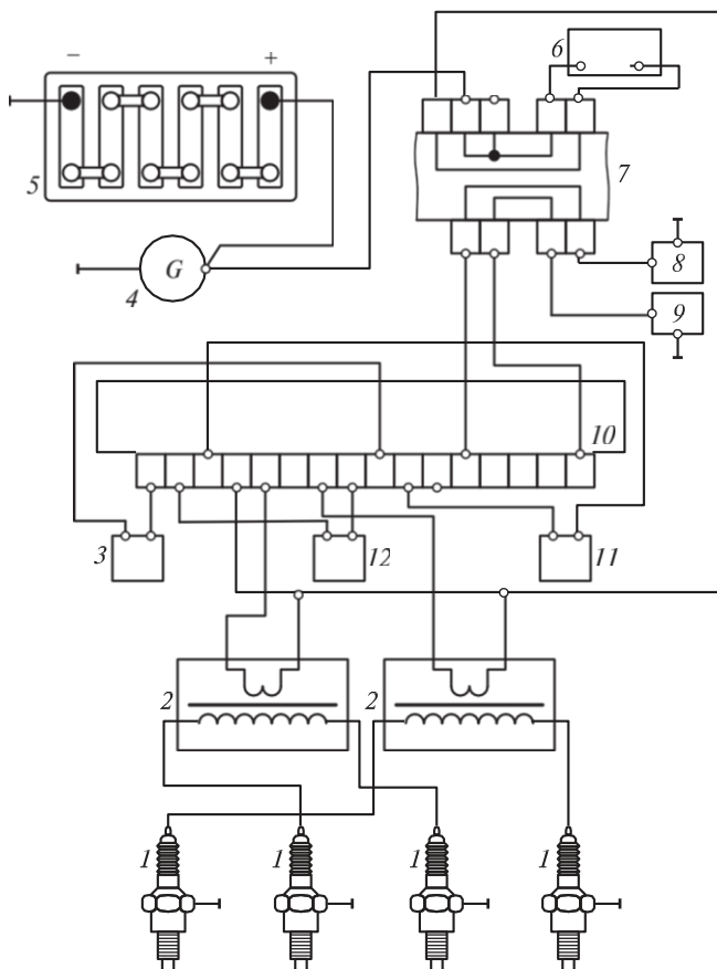
2.93 сур. Оталдыру микропроцессорлық жүйесінің құрылымдық сызбасы:
