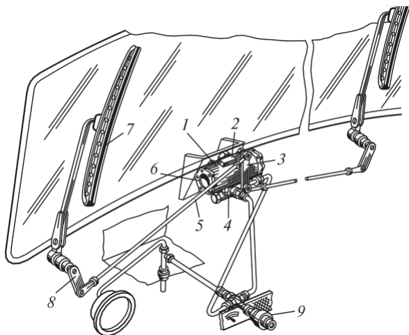
3.13 сур. ЗИЛ-431410 жүк автомобилінің пневматикалық шыны тазартқышы :
