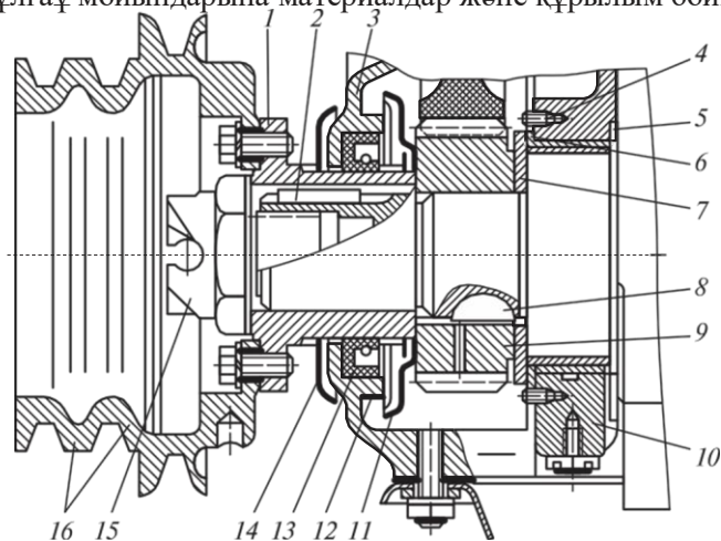
2.17 сур. Иінді біліктің өстік бекітуі және оның ұшының тығыздалуы:
