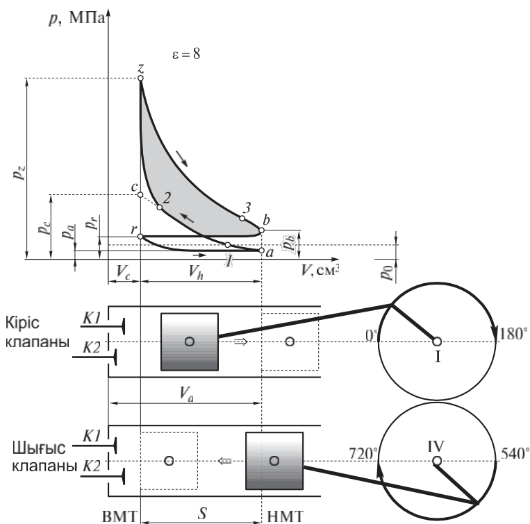
2.2. сур. Индикаторлық диаграмма қысым p — сыртқы қоспа түзуі бар іштей жану қозғалтқыштың көлемі V :
