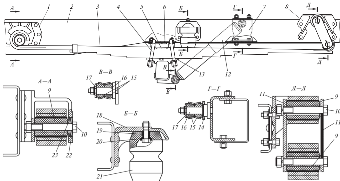
4.51. сур. ГАЗ-2752 «Соболь» автомобилінің артқы аспасы:
