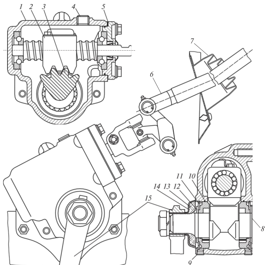
4.58. сур. ГАЗ-2752 «Соболь» автомобилінің меңгерік механизмі:
