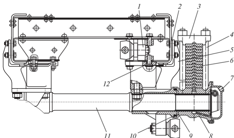
4.55. сурет. КамАЗ-65115 автомобильдерінің артқы белдемдерінің теңгергіш аспанын орнату (көлденең тілігі):
