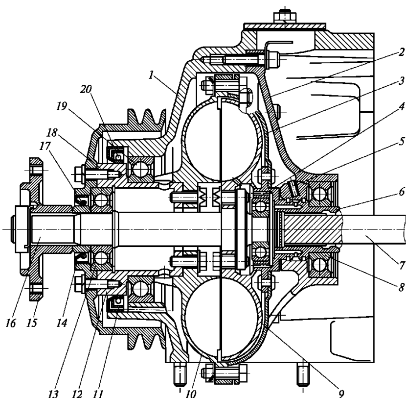
2.28 сур. Салқындатқыш жетегіндегі гидрожалғастырғыш:
