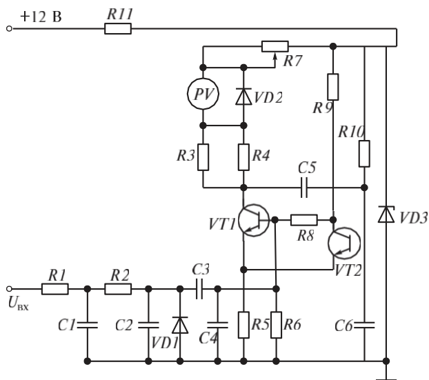
3.33 сур. Электронды тахометр сызбасы:
