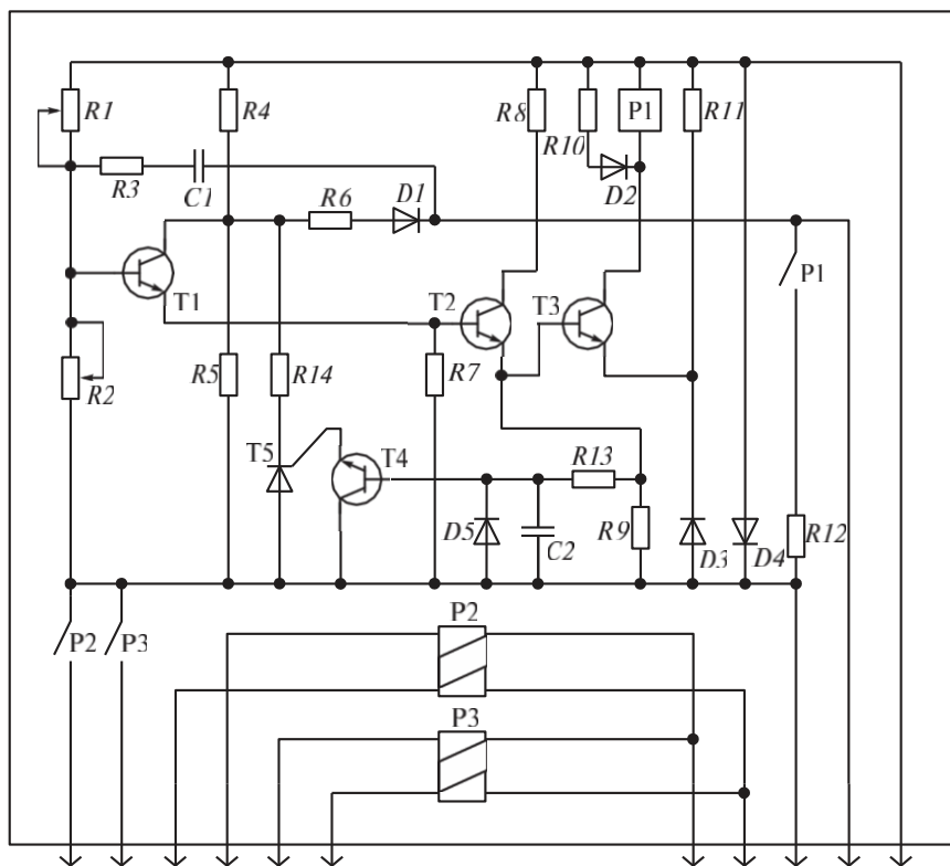
3.29 сур. КамАЗ-5320 жүк көлігінің PC951A реле-үзгішінің сызбасы: P1 —P3 — атқарушы реле; T1—T5 — транзисторлар; R1— R14 — резисторлар; D1— D5 — диодтар; C1, C2 — конденсаторлар
