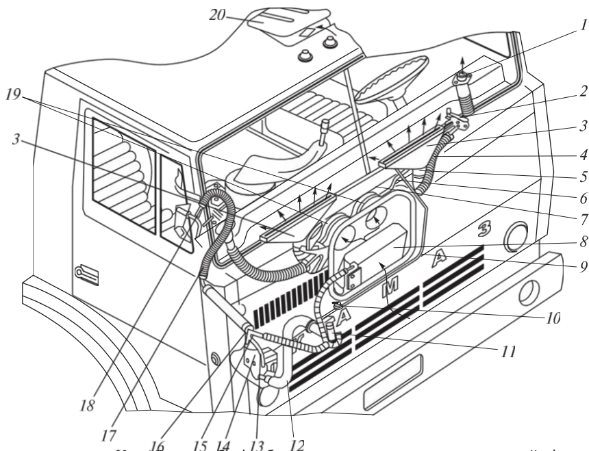
4.124 -сурет. КамАЗ автомобилі кабинасының жылыту және желдету жүйесі:
