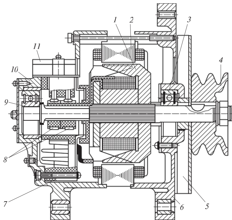
3.6 сур. КамАЗ-5320 жүк автомобилінің 65.3701 генераторы:
