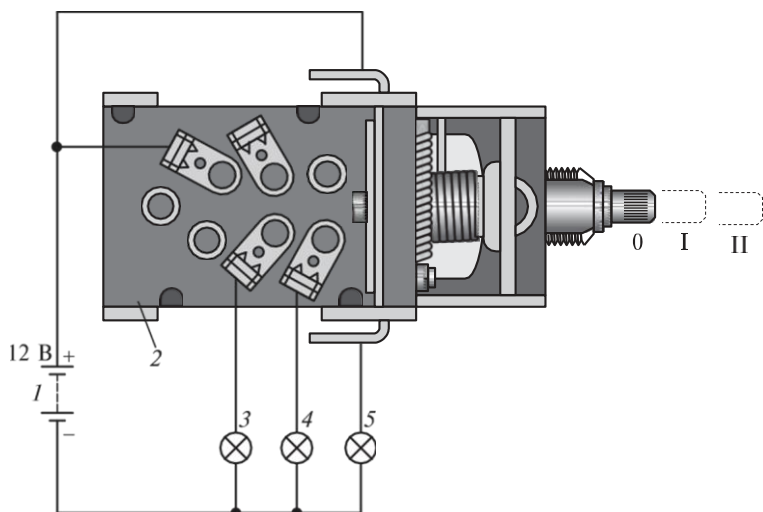
3.20 сур. Жарықтың бірыңғай орталық ауыстырып-қосқышы:
