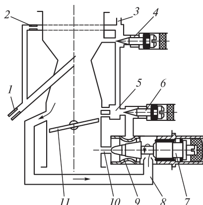
2.45 сур. Бос жүрістің автономиялы жүйесінің сызбасы:
