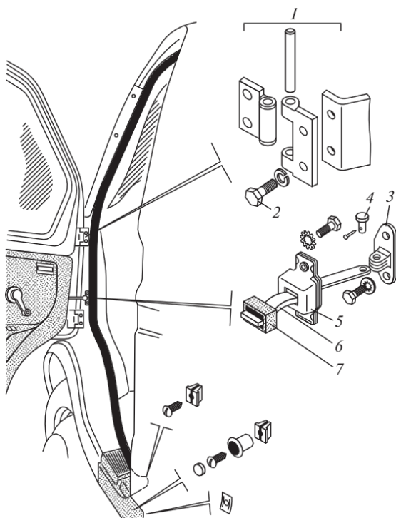
4.114 -сурет. ГАЗ-2752 «Соболь» жүк көлігінің алдыңғы есіктерінің ілмегі: 1 — ілмек; 2 — ілмекті бекіту бұрандамасы; 3 — шектеуіш тіреуіші; 4 — сұққы; 5 — шектеуіш тоқтатқышы; 6 — шектеуіш иінтірегі; 7 — буфер
