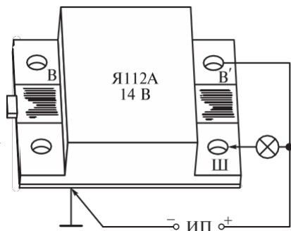
3.5 сур. Я112А кернеуінің бөлшектенбейтін реттегішінің жалпы түрі (атаулы кернеу – 14 В):
