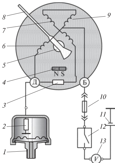
3.36 сур. 2-ші және 3-ші санаттағы ГАЗ жүк автомобильдерінің май қысымын өлшеу жүйесі:
