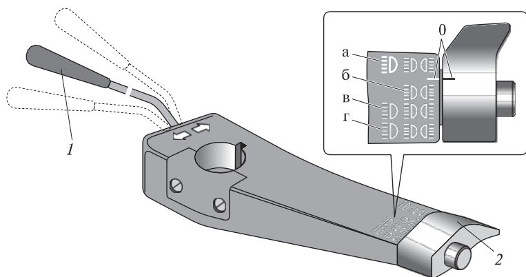
3.22 сур. КамАЗ-5320 автомобилінде габариттік шамдар мен негізгі фараларды қосу иінтірегі; 2 — шам жарығын ауыстырып-қосқыш иінтірегі; 0 — иінтіректің орналасуын өшіру; а — қысқа мерзімді дабыл үшін шамдар бекітілмеген түрде қосылады; б — алдыңғы және артқы габаритті шамдар мен нөмір белгісін жарықтандыру шамдары қосылған; в — б жағдайында, жарықтағы шам; г — б жағдайындағыдай, алыс шам жарығы
