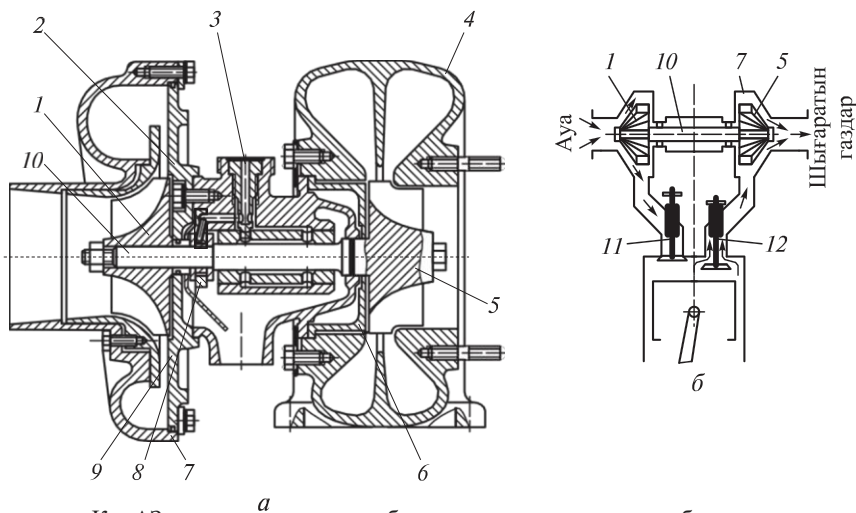
2.41 сур. КамАЗ қозғалтқышының турбо қысымды көтеру: а — турбо қысымды көтерудегі ауаны берудің құрылма жүйесі; б — жұмыс сызбасы; 1 — сығымдауыш доңгелегі; 2 — бағыттауыш аппарат; 3 — бекіткіш; 4 — турбина корпусы; 5 — турбина жоңгелегі; 6 — жылу экраны; 7, 9 — сығымдауыш корпусы; 8 — тығыздағыш сақина; 10 — ротор білігі; 11, 12 — кіріс және шығыс клапандары
