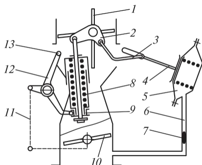
2.44 сур. Ауа жапқышының кіріс жалғама құбырындағы суық қозғалтқышты іске қосу жүйесі қондырғысының сызбасы:
