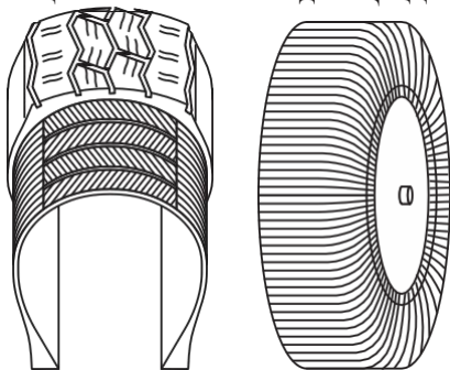
4.132-сурет. Радиалды шина: а — жалпы түрі; б — негіздің бағдарланған жіптері бар қаңқа
