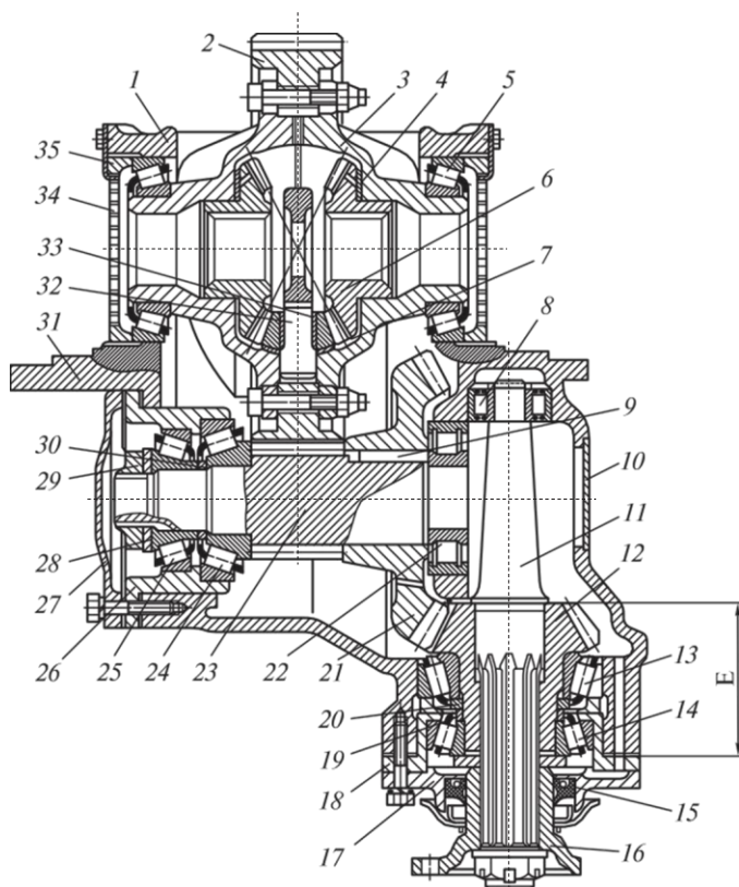
4.36 сур. Орталық конустық-цилиндр бәсеңдеткіші:
