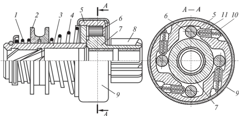
3.10 сур. Аунақша түріндегі байланыстырылмаған жүрістің муфтасы:
