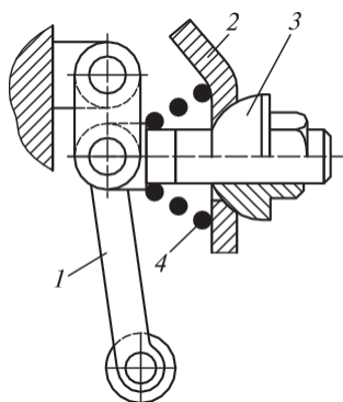
4.3 сур. Ілінісуді сөндіру иінтірегі жетегінің сызбасы:
