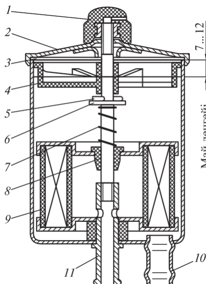
4.65. сурет. ГАЗ-2752 «Со- боль» және ГАЗ-33021 «Газель» автомобильдерінің меңгерік басқару гидрокүшейткішінің құбішесі: 1 — қалпақшалы сомын; 2 — қақпақ; 3 — төсем; 4 — торлы сүзгі; 5 — сірге; 6 — тығырық; 7 — серпіше; 8 — конустық тығыздағыш тығырық; 9 — қағаз сүзгіш элементі; 10 — майды сорғыға беретін жалғама құбыр; II — майды таратқыш корпусынан күбішеге әкелетін жалғама құбыр
