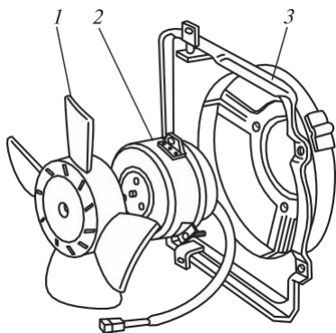
2.27 сур. Салқындатқыштың электр жетегі:
