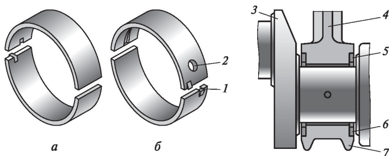
2.15 сур. Жартылай цилиндрлік жінішке ұабырғалы ішектер: а — бұлғақтық; б — іргелі; в — жинаудағы бұлғақты ішек; 1 — бекітілген дөңес; 2 — майланған саңылауы; 3 иінді білік; 4 — бұлғақ; 5, 6 — жартылай цилиндрдік ішектер; 7 — бұлғақ қақпасы
