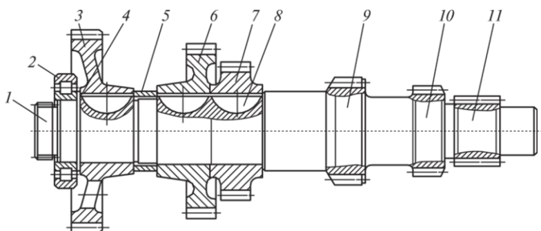
4.16 сур. КамАЗ автомобильдерінің аралық білігі:
