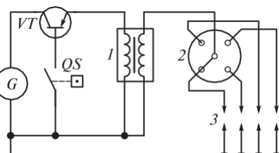
2.90 сур. Оталдырудың түйіспелі транзисторлы жүйесінің сызбасы: 1 —оталдыру орамы; 2 —тараушы; 3 — ұшқын білтелері; G — энергия көзі (генератор); VT — транзистор; QS — бөлгіш
