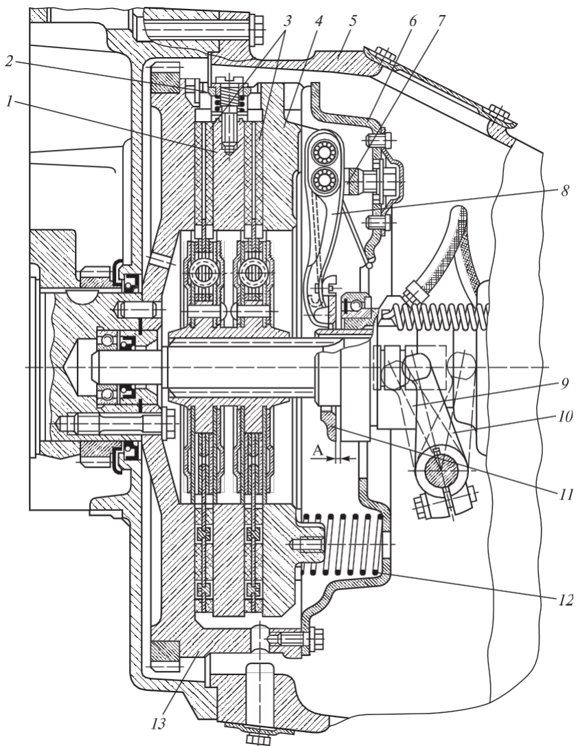
4.5 сур. КамАЗ-5301 екі дискілі ілінісуі:
