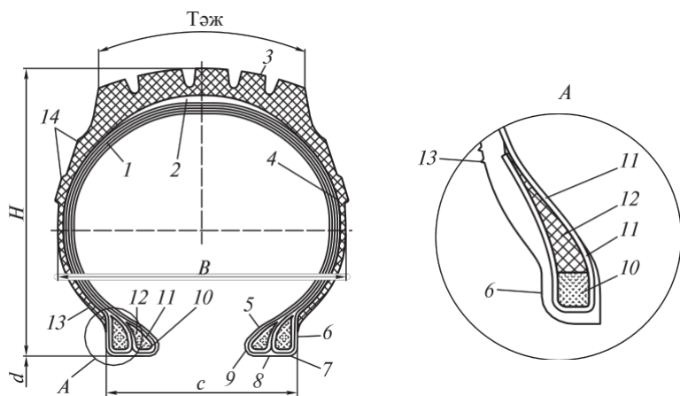
4.130 -сурет. Заманауи шина:
