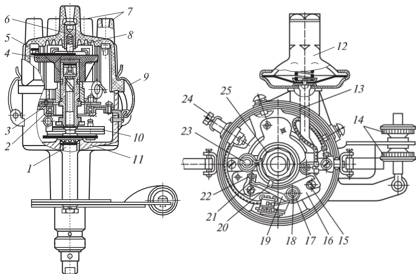
2.86 сур. Оталдырудың үзгіш-таратушысы:
