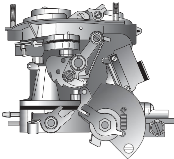
Сурет. 2.52. Дроссельдерді басқару драйвері
