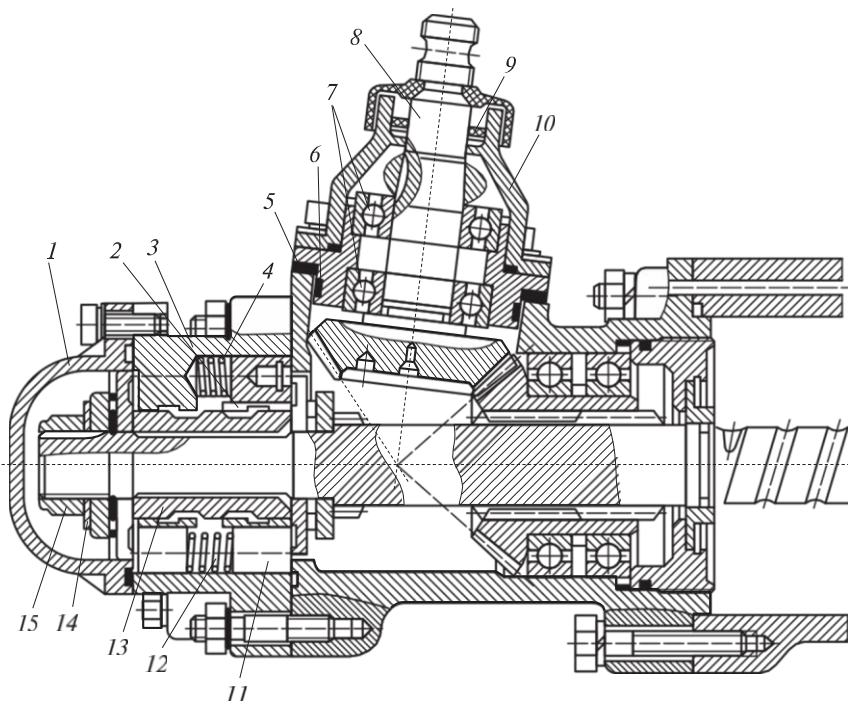
4.72. сурет. КамАЗ автомобильдерінің осьтік типті бөліп таратқышы бар ыаракшы құрылғысы:
