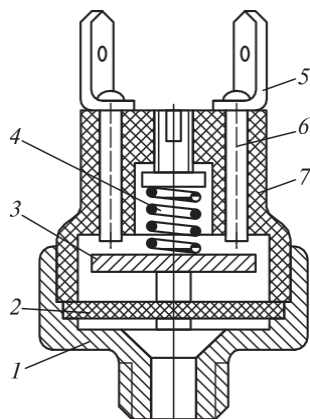
3.26 сур. Тоқта-дабыл шамын қосу пневматикалық қадағасы
