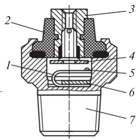
3.35 сур. Салқындатқыш сұйықтығының апатты қызып кету дабылқаққышының қадағасы:
