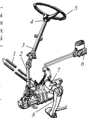
4.69. сурет. КамАЗ автомобильдерінің меңгерік басқаруының жалпы құрастырымы: 1 — май радиаторы; 2, 4 — біліктер; 3 — басқару бағанасы; 5 — меңгерік дөңгелегі; 6 — меңгерік гидрокүшейткішінің сорғысы; 7 — меңгерік механизм; 8 — сирақ
