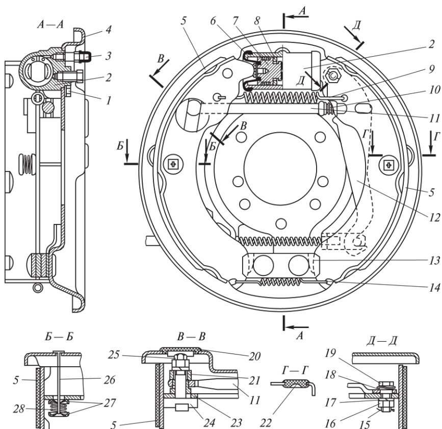
4.79 -сурет. ГАЗ-2752 «Соболь» және ГАЗ-3302 «Газель» автомобильдерінің барабан тежеуіш тетіктері:
