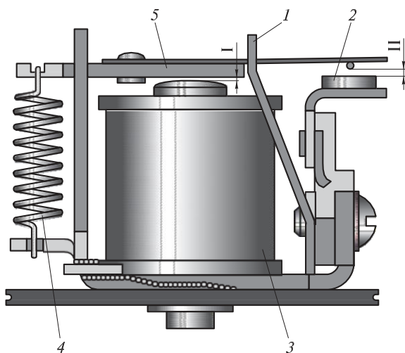
3.28 сур. Бұрылудың жарық көрсеткіштерінің электр магнитті релесі: 1 — экірдің жүрісін шектегіші; 2 — байланыс; 3 — катушка; 4 — тығынжыл; 5 — жыжымалы байланыс (экір); I — жүрекше мен экір арасындағы саңылау; II — байланыстар арасындағы саңылау
