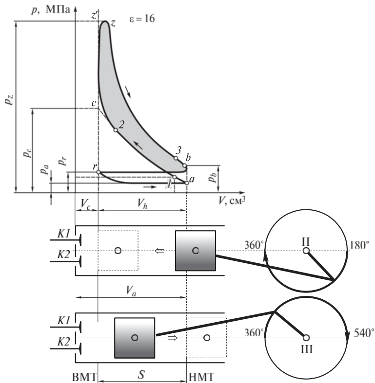
2.3 .сур. Индикаторлық диаграмма қысым p — дизель V көлемі: 2.2 сур. белгілер тура сондай; II, III — қозғалтқыштың жұмыс ырғақтары (сығылу және жұмыс жүрісі)
