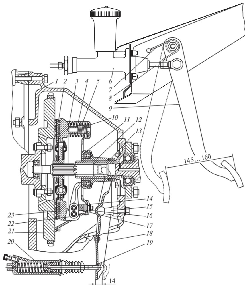
4.4 сур. ГАЗавтомобилінің ілінісуі:
