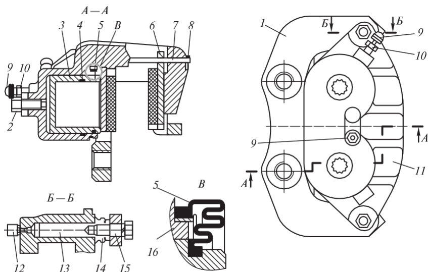
482 сур. ЗИЛ-5301 автомобилінің алдыңғы дөңгелектерінің дискілі тежеуіші:
