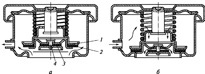
224 сур. Құйғыш қылтаның тығынындағы бу ауа клапаны жұмысының сызбасы: а — бу клапаны әрекетінің кезі; б — ауа клапаны әрекетінің кезі; 1 — бу клапаны; 2, 3 — тығыздауыш төсемшелер; 4 — ауа клапаны
