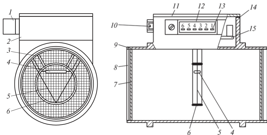
2.68 сур. Термоанемометрикалық бергіш:
