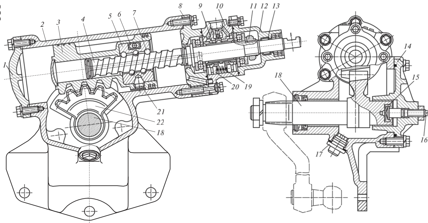
Сурет. 4.68. ZIL-5301 автокөлігінің руль механизмі:
