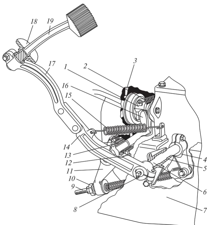
4.8 сур. ЗИЛ-5301 автомобилі ілінісуін басқарудың механикалық жетегі:
