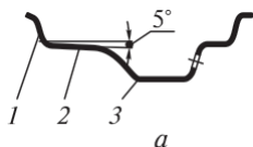
4.126 -сурет. Жүк автомобилі дөңгелегінің тұтас тоғыны:
