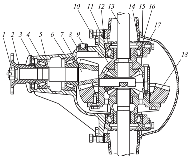
4.32 сур. ГАЗ-2752 «Соболь» автомобилінің артқы жетекші белдігінің ортаңғы бөлігі:
