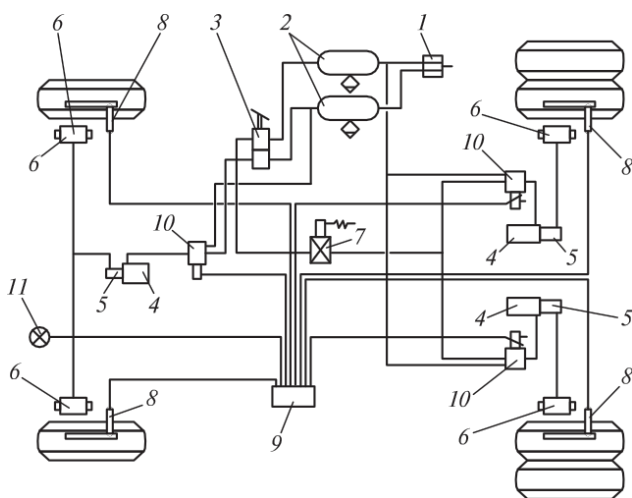
481 сур. ЗИЛ-5301 «Бычок» шағын жүк автомобилінің тежеуіш басқару жетегінің сызбасы:
