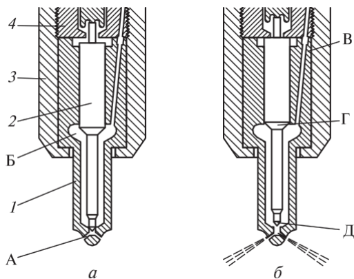
2.84 сур. Тығын инесінің пішіні:
