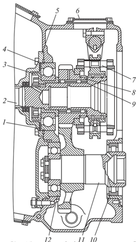
4.27 сур. КамАЗ-5410 ершікті тартқышындағы бөлгіш:
