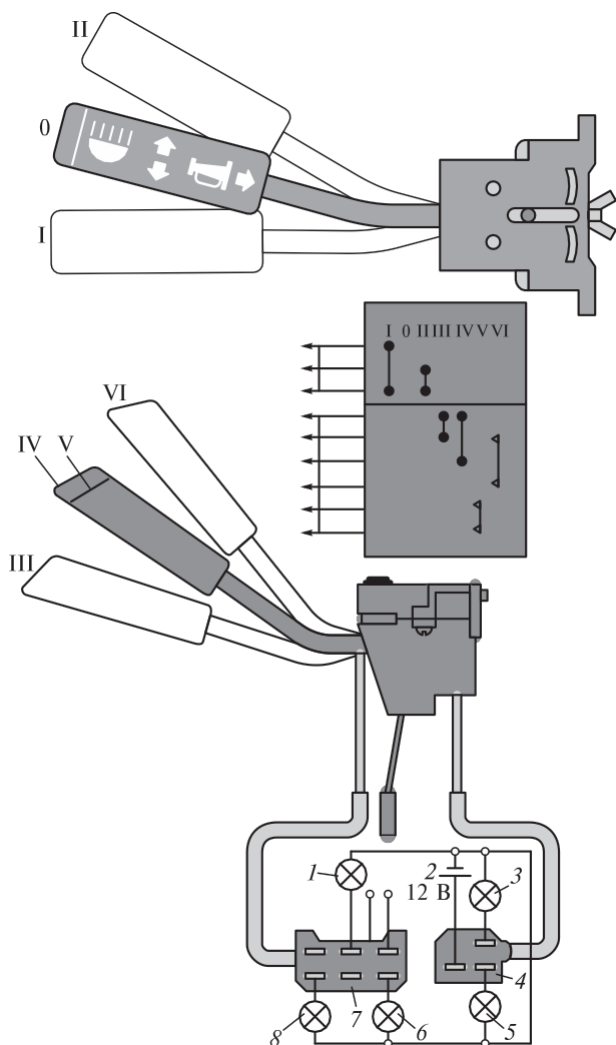
3.21 сур. Жақыннан алысқа ауыстырып қосқыш сызбасы:
