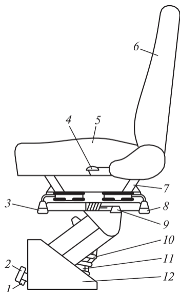
4.115 -сурет. ГАЗавтомобилі жүргізушісі орындығының құрылымы:
