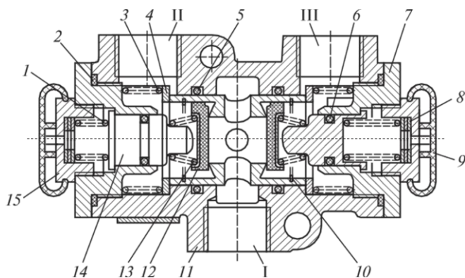
4.103 -сурет. Қосарланған қорғағыш клапан:
