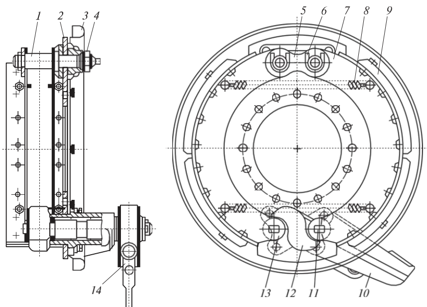
4.86 сур. КамАЗ автокөлігінің тежеуіш тетігі:
