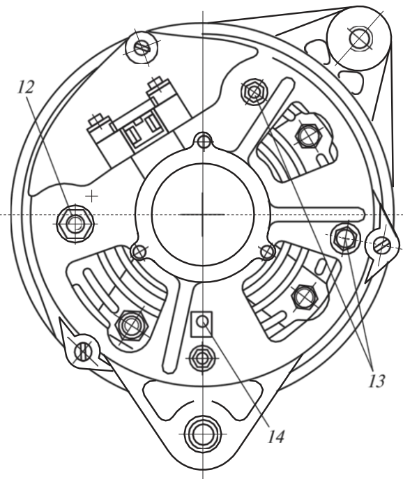
3.6 сур. КамАЗ-5320 жүк автомобилінің 65.3701 генераторы:
