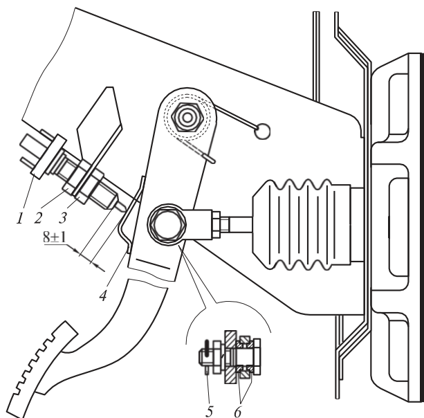
3.25 сур. ГАЗ жүк автомобильдеріндегі тоқта-дабыл шамдарын қосқыш; 1 — тежегіш жарығы дабылын қосқыш; 2, 3 — сомын; 4 — басқыштың табанды алаңы; 5 — сірге; 6 — пластмасс төлкелер
