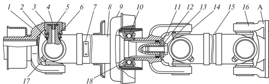
4.31 сур. ГАЗ-2752 «Соболь» автомобилінің кардан берілісі:
