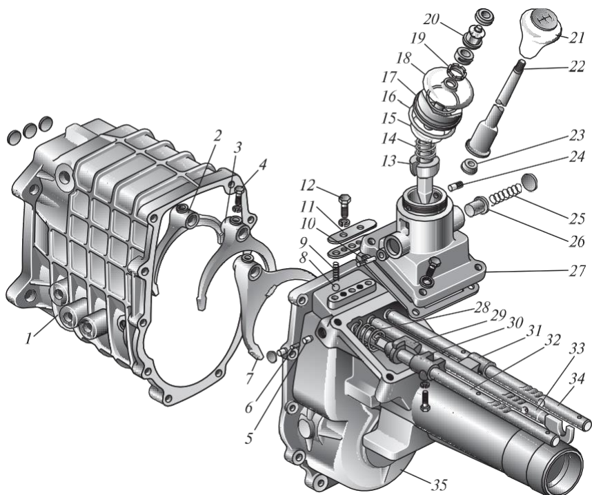
4.13 сур. ГАЗ-2752 «Соболь» автомобилі берілісін ауыстыру механизмі:
