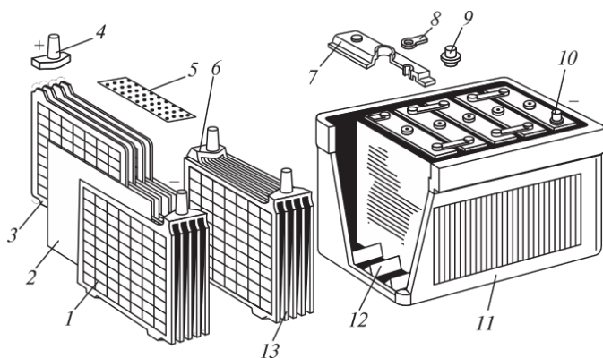
3.1 сур. 12 В кернеулі типтік аккумулятор батареясы:
