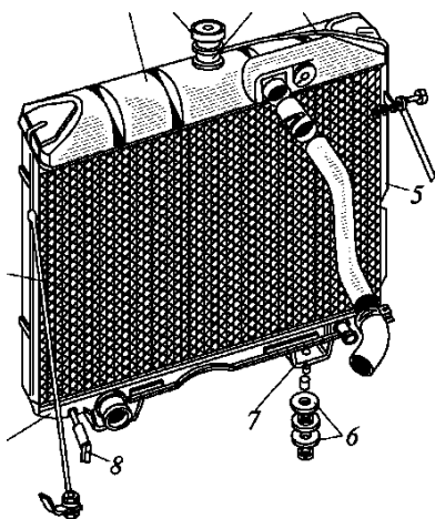
2.23 сур. Жүк автомобильдің радиаторы өзінің негізгі элементтерімен жинақтастыруда:
