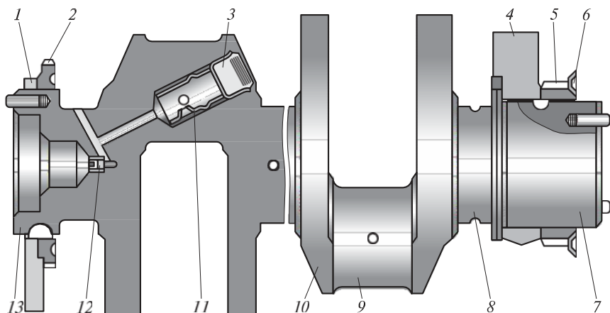
2.16 сур. Иінді білік:
