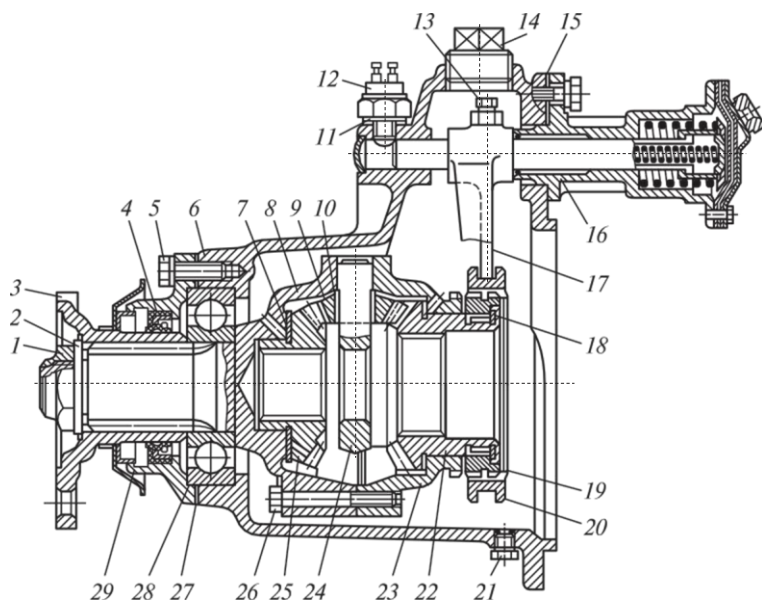
4.37 сур. КамАЗ-5320 автомобилінің ось аралық дифференциалы:
