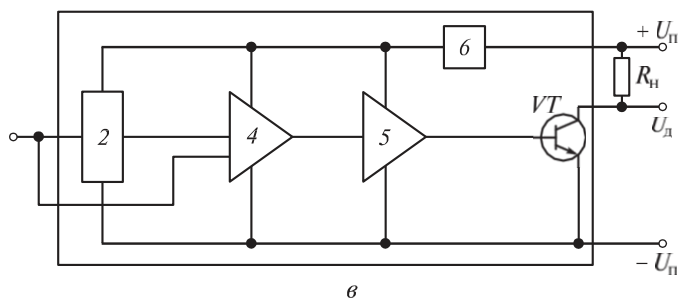
2.92 сур. Холл бергішін қолдана отырып бастапқы тізбектің үзілуінің түйіспесіз жүйесінің сызбасы :
