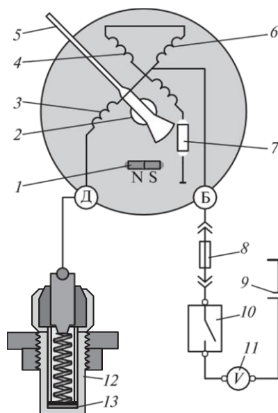
3.34 сур. ГАЗ жүк автомобильдері қозғалтқышының салқындатқыш сұйықтығы температурасын өлшеу жүйесі:
