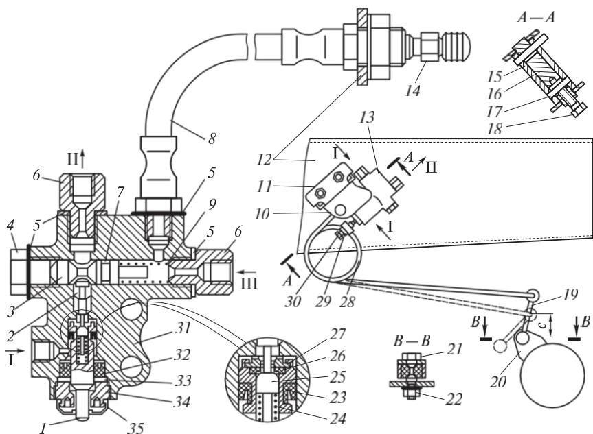
4.76 -сурет. ГАЗ-2752 «Соболь» автомобилінің сөндіру тетігі бар тежеу күші реттегіші:
