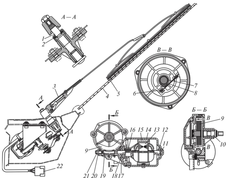
3.12 сур. Электр шыны тазартқыш:
