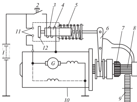
3.8 сур. Стартердің, оның қуат жүйесінің және иінді біліктің айналу жиілігінің жалпы сызбасы:
