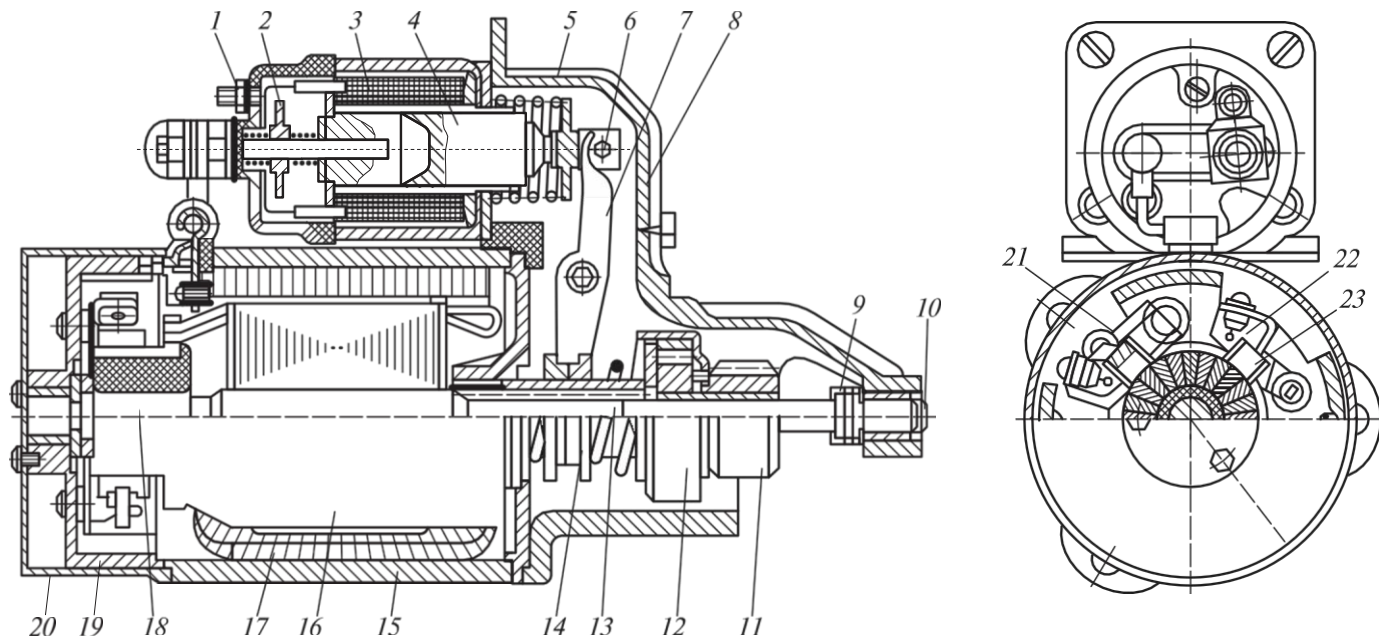
3.9 сур. ЗИЛ-5301 жүк автомобилінің 20.3708 стартері:
