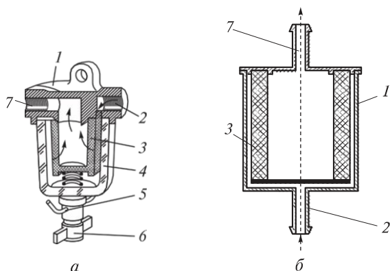
2.39 сур. Ақтап тазалаудың отын сүзгілері: а — бөлшектегі; б — бөшкеусіз; 1 — корпус; 2 — кіріс саңылауы; 3 — сүзгілеуші элемент; 4 — алмалы пластмассалық стакан-тұндырғыш; 5 — ұстағыш; 6 — бекіту сомыны; → — отын қозғалысы
