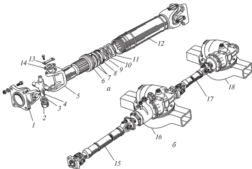
4.30 сур. КамАЗ-5320 автомобилінің қардан берілісі: а — екі ойма кілттекті қардан берілісінің құрылымы; б — жетекші белдіктердің жетегі; 1 — фланец-аша; 2 — инелі мойынтірек; 3 — тығыздағыш шығыршық; 4 — айкастырма; 5 — аша; 6 — сомын (шеңбер); 7, 9, 11 — тілінген тығырық; 8 — киіз шығыршық; 10 — резенкелі шығыршық; 12 — қардан білігі; 13 — тоқтатқыш тілім; 14 — жапқыш тілім; 15 — орта жетекші белдіктің жетекші тегершігінің қардан білігі; 16 — орта жетекші белдік; 17 — артқы жетекші белдік жетегінің қардан білігі; 18 — артқы жетекші белдік
