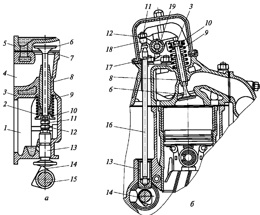
220 сур. Үйлестіруші біліктің төменгі орналасуында клапандардың жетегі: a — клапанның төменгі орналасуы; б — клапанның жоғары орналасуы; 1 — блок-картердің ішкі қуысы; 2 — блок-картер; 3 — ұнтақтар; 4 — коллектор; 5 — цилиндрлер блогының бастиегі; 6 — клапан; 7 — ер; 8 — клапан бағыттаушысы; 9 — серіппе; 10 — тарель; 11 — реттеуші бұрама; 12 — қарсысомын 13 — итергіш; 14 — жұдырықша; 15 — үйлестіруші білік; 16 — итергіш қарнағы; 17 — иінағаштың тіреу өсі; 18 — иінағаш; 19 — иінағаш өсі
