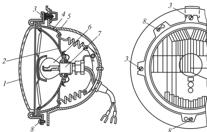
3.17 сур. Дөңгелек фара:
