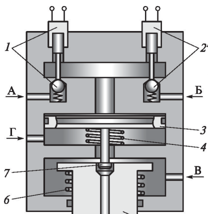
сур. 4.85. ЗИЛ-5301 автомобилінің АБС модуляторының қағидалық сұлбасы: 1, 2 — электромагниттік клапандар; 3 — қадағалаушы піспек; 4, 6 — серіппелер; 5 — атмосфералық клапан ершігі; 7 — кіру және атмосфералық клапандар корпусы; А, Б, В, Г, Д — модуляторды тиісінше тежегіш кранға, атмосфераға, ауа баллонына, тежегіш камерасының жұмыс қуысына және де соңында тежегіш камераны модулятор арқылы атмосфераға қосатын өңештер
