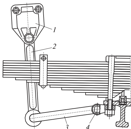
4.50. сурет. КамАЗ-53212, -53222, -54112 және -54122 автомобильдерінің алдыңғы аспасының көлденең тұрақтылығын тұрақтандырғыш: 1 — тұрақтандырғыштың тіреуіші; 2 — тірек; 3 — қарнак; 4 — тұрақтандырғыштың төменгі тіреуіші
