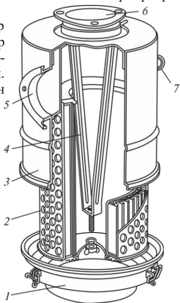
2.40 сур. КамАЗ қозғалтқыштарындағы ауаны тазартуға арналған қағаз алмалы сүзгісі: 1 — қақпақ; 2 — сүзілеуші элемент
