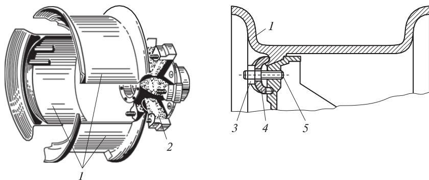
4.127 -сурет. Дискісіз дөңгелек:
