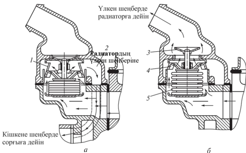
2.30 сур. Сильфонды түрлі термостат жұмысының сызбасы:
