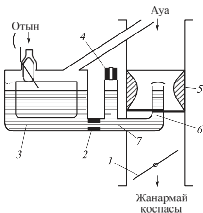
2.43 сур. Өтемді құдығы бар карбюратор:
