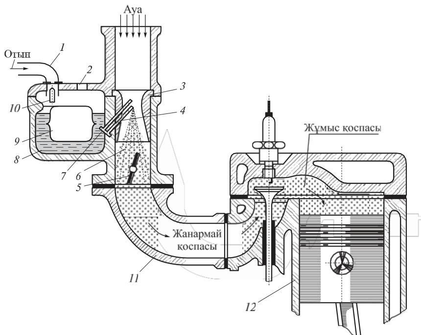
2.42 сур. Қарапайым карбюратор жұмысының сызбасы:
