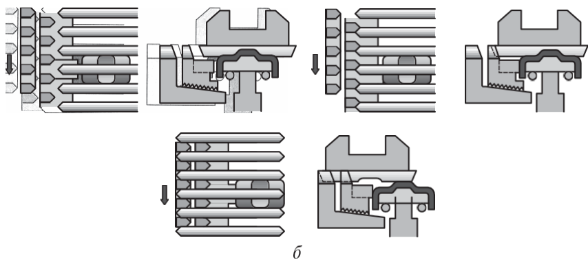
4.12 сур. Инерциялық типті муфталық синхрондауыш: а — құрылғы; б — жұмыс қағидасы; 1 — бастапқы білік; 2 — бұғаттаушы шығыршық; 3 — сухарь; 4 — қосылудың тісті муфтасы; 5 — серіппе; 6 — күшпек; 7 — III берілістің тегершігі; >=> — айналым бағыты
