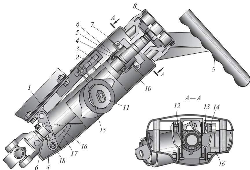
4.56. сурет. ГАЗ-2752 «Соболь» автомобилінің меңгерік механизмінің жетегі : 1, 17 — тіреуіштер; 2 — сектор; 3 — басқару бағанасының құбыры; 4 — мойынтірек; 5 — мойынтіректің төлкесі; 6 — тоқтатқыш сақина; 7 — үстінгі қаптама; 8 — жапсырма; 9 — меңгерік дөңгелек; 10 — төменгі қаптама; 11 — тұтандыру тетігі; 12 — сомын; 13 — тіректі тығырық; 14 — бұрандама; 15 — қапсырма; 16 — басқару бағанасының қалпын бекіту иінтірегі; 18 — иінтірек
