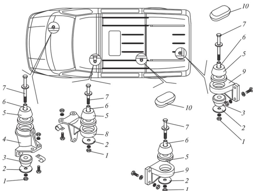
4113 -сурет. ГАЗ-2752 «Соболь» жүк автокөлігі шанағының тіректері: 1 — сомын; 2 — тығырық; 3, 5 — жастықтар; 4, 8, 9 — тіреуіштер; 6 — керме төлке; 7 — бұранда; 10 — бітеуіш
