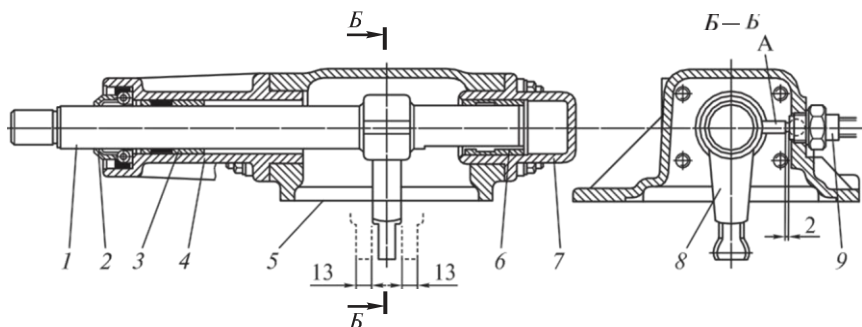
4.23 сур. КамАЗ автомобильдері берілісін ауыстыру иінтірегінің тірегі:
