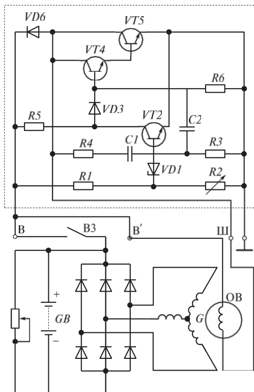
3.4 сур. Я112А кернеу реттегішінің сызбасы:
