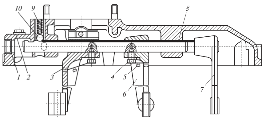
4.20 сур. КамАЗ автомобильдерінің берілісті ауыстыру механизмі:
