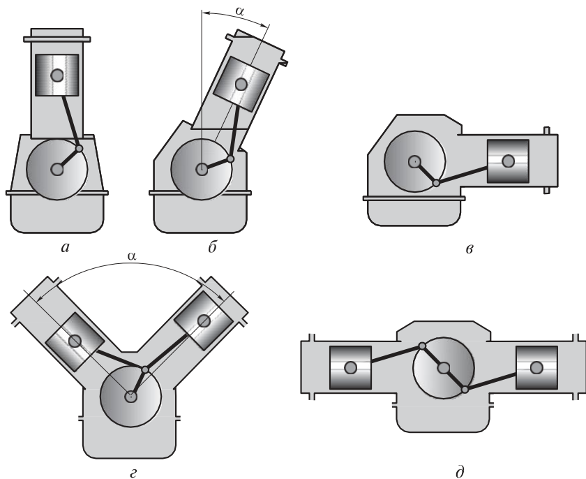
2.4 .сур. Жүк автомобильдер қозғалтқыштарында цилиндрлерорналасуының ықтимал сызбалары:
