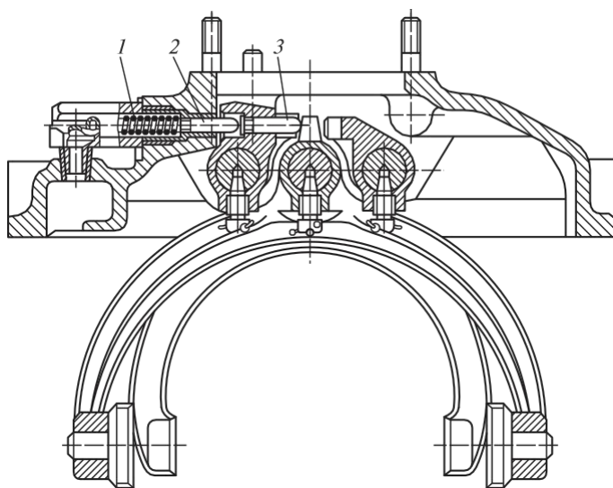
4.22 сур. КамАЗ автомобильдері берілісін ауыстыру механизмінің сақтандырғышы:
