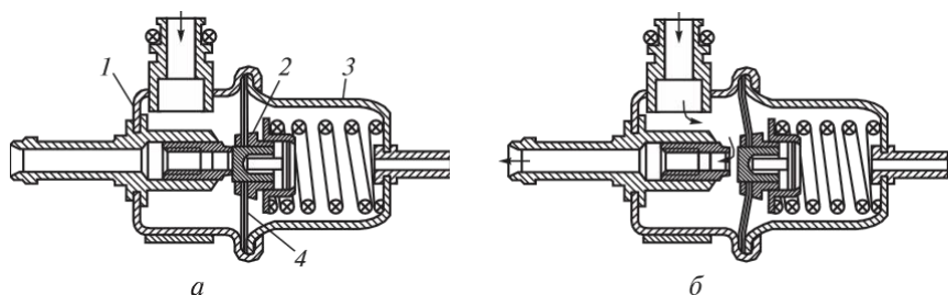
2.61 сур. Қысым реттегіші:
