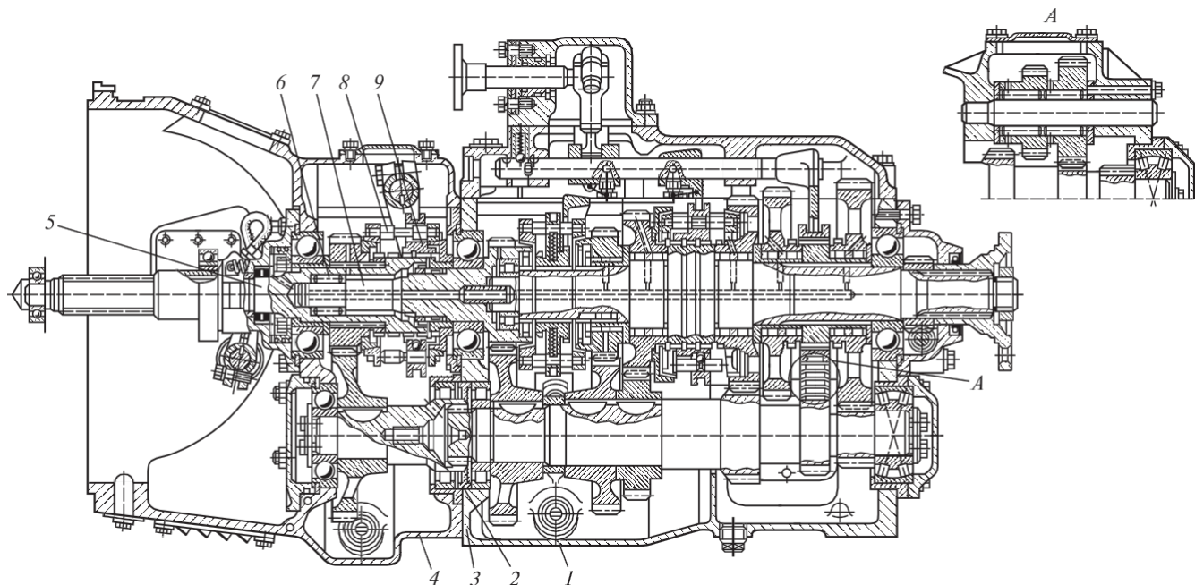
4.29 сур. Бөлгішті беріліс қорабының жалпы сипаты:
