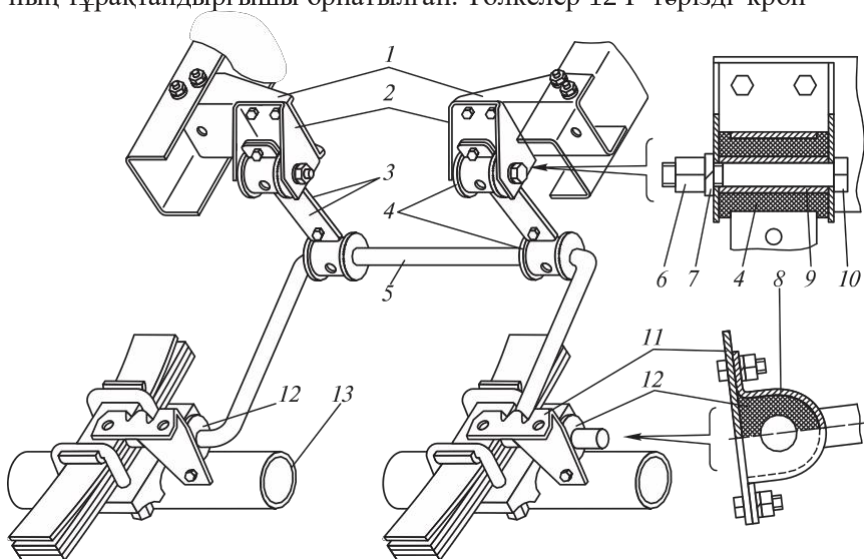
4.52 сур. ГАЗ-2752 «Соболь» автомобилінің артқы аспасының көлденең орнықтылығының тұрақтандырғышы:
