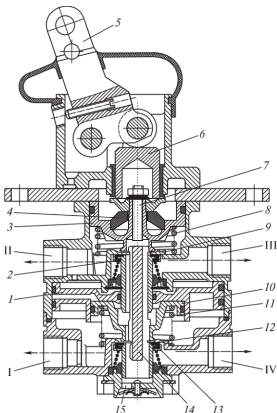
4.105 -сурет. КамАЗ автокөліктерінің Г100-3514000 екі секциялы тежегіш шүмегі: 1 — тездеткіш піспек; 2, 13 — жоғарғы және төменгі клапандар; 3, 10 — қадағалау піспектері; 4 — тығырық; 5 — иінтірек; 6 — итергіш; 7 — тірек түйреуіш; 8, 11 — қадағалау піспегінің серіппелері; 9, 12 — клапан ершіктері; 14 — бағыттағыш өзек; 15 — атмосфераға шығыс; I — IV — қуыстар
