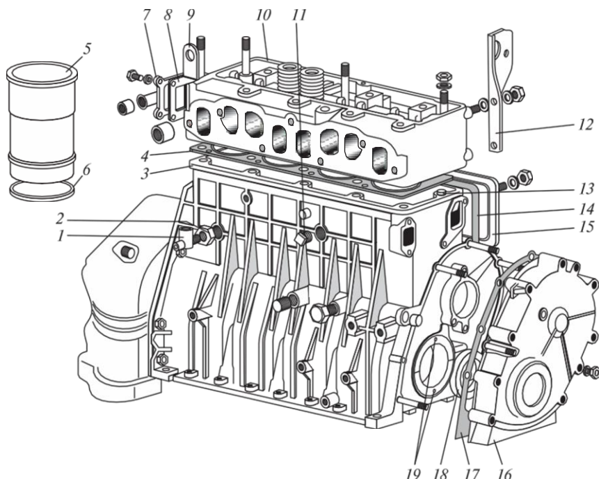
27. сур. ГАЗ-33021 қатарлы қозғалтқышты автомобильдің цилиндрлер блогы және цилиндрлер бастиегі:
