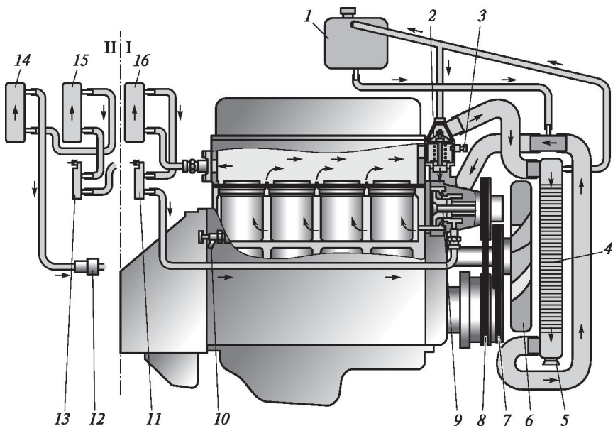
2.22 сур. Қозғалтқышты сұйықтық салқyndату жүйесі :
