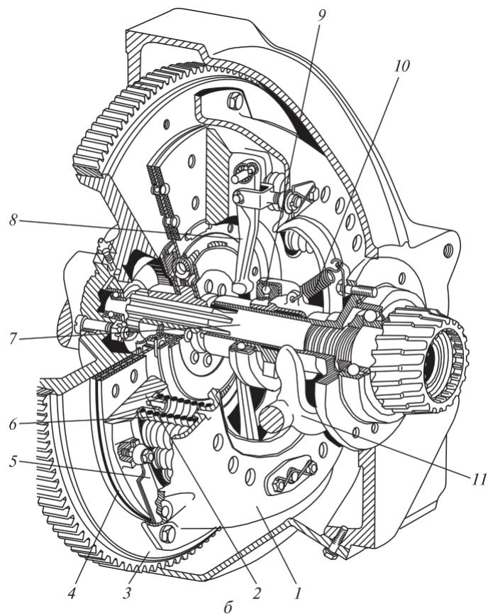
4.1 сур. Бір дискілі үйкелісті ілінісудің сызбасы (а) және конструкциялық орындалуы (б): 1 — қаптама; 2 — қысқыш диск; 3 — сермер; 4 — жетектегі диск; 5 — топса; 6 — қысқыш серіппе; 7 — БҚ жетекші білігі (шығыс білік); 8 — ілінісуді сөндіру иінтірегі; 9 — ілінісуді сөндіру мойынтірегі; 10, 13 — тарту серіппелері; 11 — аша, 12 — басқыш; 14 — күш
