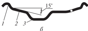
4.126 -сурет. Жүк автомобилі дөңгелегінің тұтас тоғыны:
