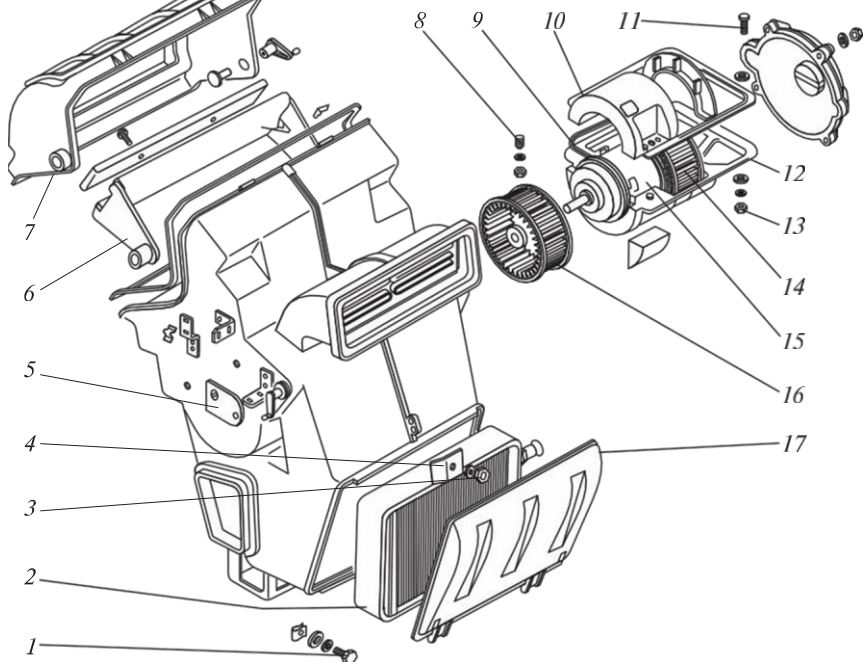
4.121 -сурет. ГАЗ-3302 «Газель» және ГАЗ-2752 «Соболь» автомобильдерінің жылытқышы:
