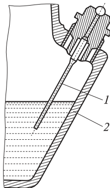
4.26 сур. Май деңгейі көрсеткіші қондырғысы:
