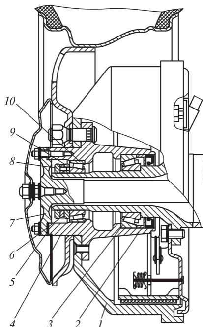
4.128 -сурет. Діскінің бекіту тесіктеріндегі конусты жүзді күпшектерде дөңгелектерді орталықтау:
