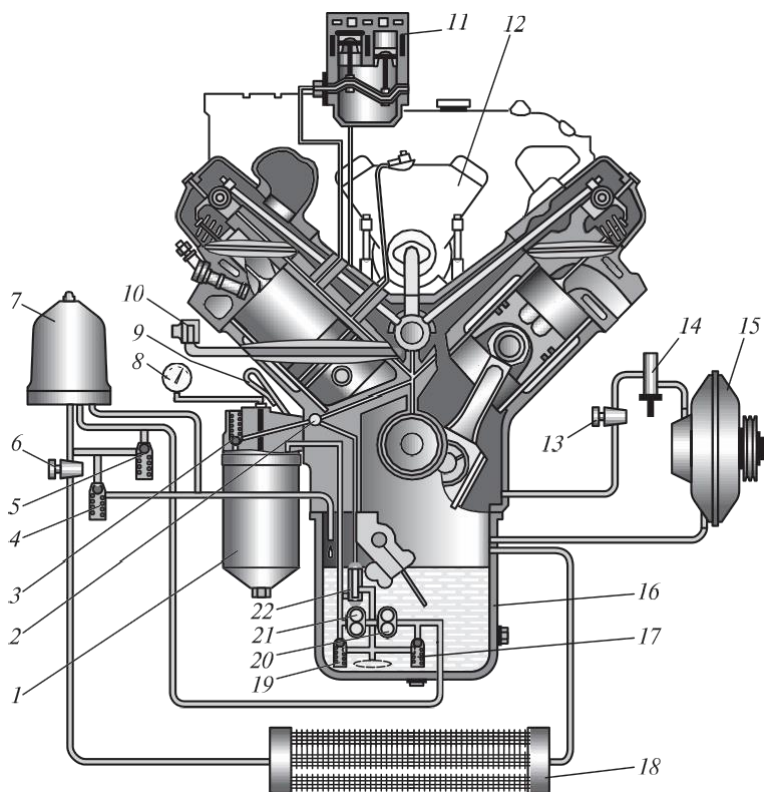
2.36 сур. КамАЗ-740 қозғалтқышы майды тазалау құрамдастырылған жүйесі:
