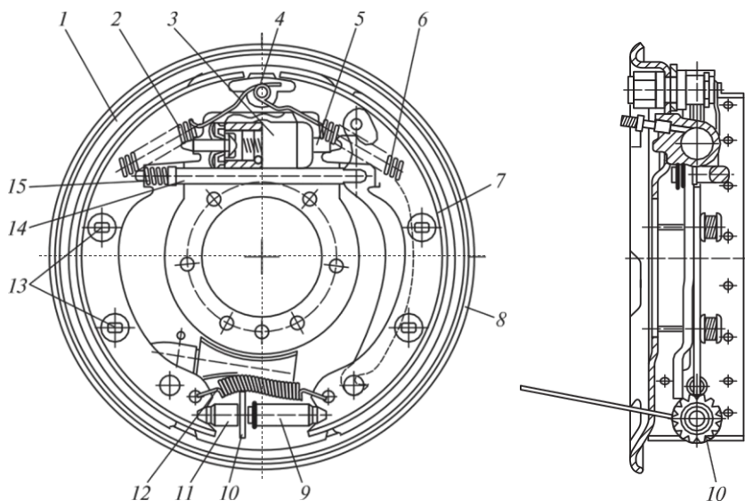
483 сур. ЗИЛ-5301 автомобилінің артқы дөңгелектерінің тежеуіш механизмі:
