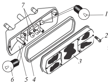
3.19 сур. ЗИЛ-5301 автомобилінің артқы блок-шамы:
