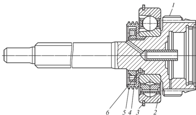
4.15 сур. КамАЗ автомобилінің БҚ бастапқы білігі:
