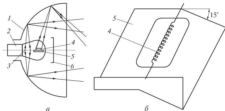
3.16 сур. Сыртқы жарықтандыру фаралары: а — жақын және алыс жарық (CR) фаралары; б — шамдағы қызу жібін орнату сызбасы; 1 — шағылдырғыш; 2 — шам; 3 — алыс жарық жібі; 4 — жақын жарық жібі; 5 — төменгі сәулелер экраны; 6 — тура сәулелер экраны
