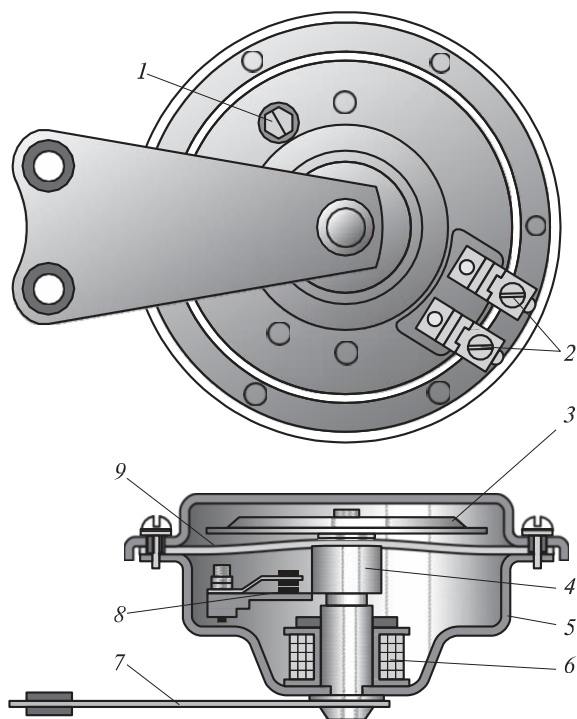
3.30 сур. Шулы электр магнит тербелісті дабыл беру:
