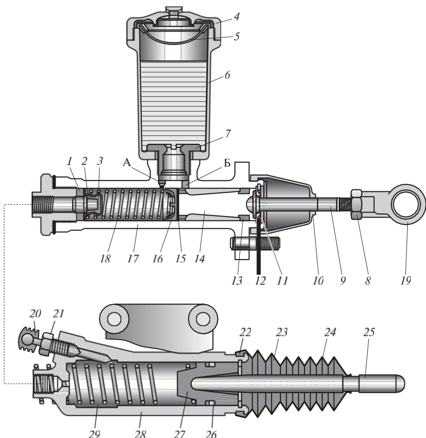
4.9 сур. Басты және жұмыс цилиндрлердің құрылымы:
