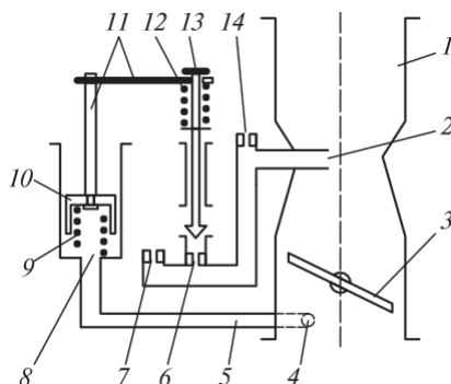
2.49 сур. Арнайы піспектің сояуышы бар экономайзер:
