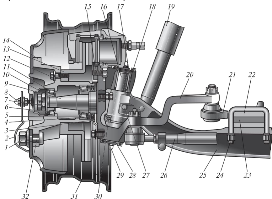
4.43. сурет. ГАЗ-3302 автомобилінің алдыңғы аспасы:
