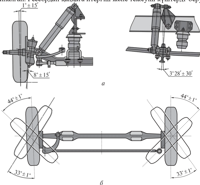
4.46. сурет. ГАЗ-3302 «Газель» автомобилінің жетектегі белдемі: а — рессорды, амортизаторды және резеңке буферді орнату; б — алдыңғы белдем арқалығының түрі
