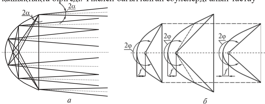
3.15 сур. Параболоидті шағылдырғыш: а — алыс және жақын сәулелерді қалыптастыру сызбасы; б — шағылдырғыштың болжамды пішіндері; 2\alpha — сәуленісейілткіш бұрышы; 2\phi — шағылдырғышты қысу бұрышы; f — фокусты қашықтық
