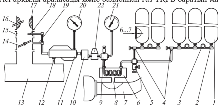
2.54 сур. Газ балонды қондырғыдан қуат алатын қозғалтқыштың қоректендіру жүйесі:
