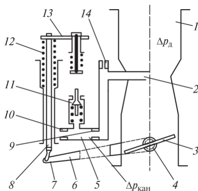
2.48 сур. Кедергі ашылуының механикалық жүйелі экономайзеры: 1 — карбюратордың кіріс жалғама құбыры; 2 — бүріккіш; 3 — кедергі қалқаны; 4 — кедергі қалқанының өсі; 5 — жиклераралық қуыс; 6 — тетік; 7 — тіркелгіш түйін; 8 — сояуыш; 9, 10 — отын жиклерлері; 11 — экономайзер клапаны; 12 — серіппе; 13 — серіппелі сояуыш бар денгейі; 14 — ауа жиклері; \Delta p_d — кедергі қалқанының астындағы сөйіліту; \Delta p_{кан} — сөйіліту
