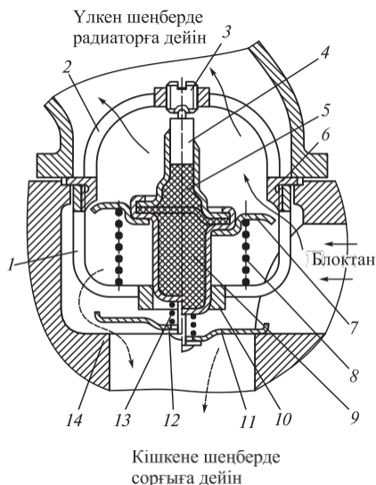
2.31 сур. Қатты толтырғышы бар термостат жұмысының сызбасы:
