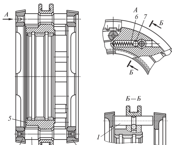
4.18 сур. КамАЗ автомобильдерінің II және III берілісінің синхрондауышы: 1 — фиксатор сұққысы; 2 — II берілістің фрикциялық шығыршығы; 3 — бұғаттаушы сұққы; 4 — III берілістің фрикциялық шығыршығы; 5 — синхрондауыш күймешесі; 6 — фиксатор серіппесі; 7 — кіші шар
