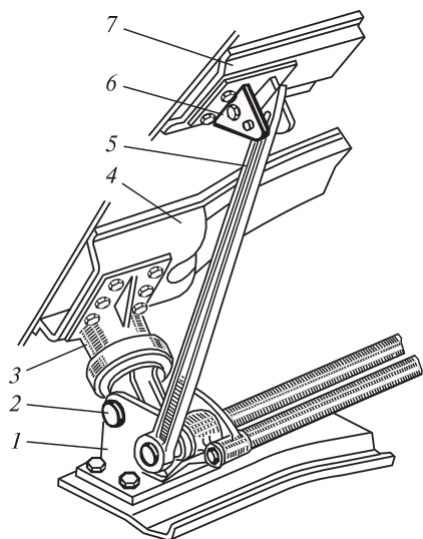
4117 -сурет. Передняя опора кабины:
