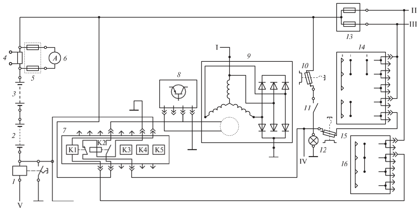
3.39 сур. КамАЗ-5320 жүк автомобилінің электр қамту жүйесінің сызбасы:
