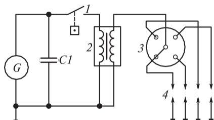
2.85 сур. Қоректенудің үзілетін түйісу жүйесімен бірге оталдыру жүйесі: 1 — үзгіш; 2 — оталдыру орамы; 3 — оталдыру таратушысы; 4 — ұшқын оталдыру білтелері; G — энергия көзі (генератор немесе аккумулятор батареясы); CI — конденсатор
