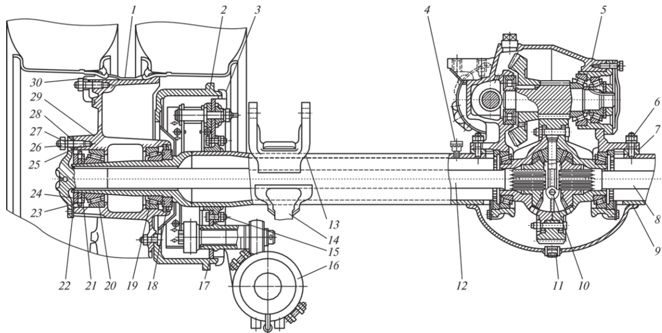
4.35 сур. КамАЗ-5320 автомобилінің артқы белдігі:
