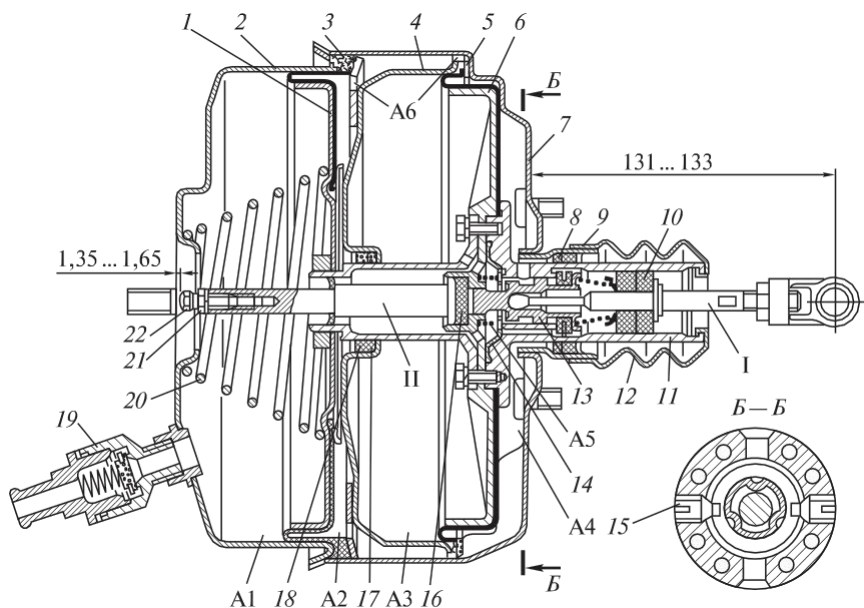
Рис. 4.74. Вакуум күшейткіші:
