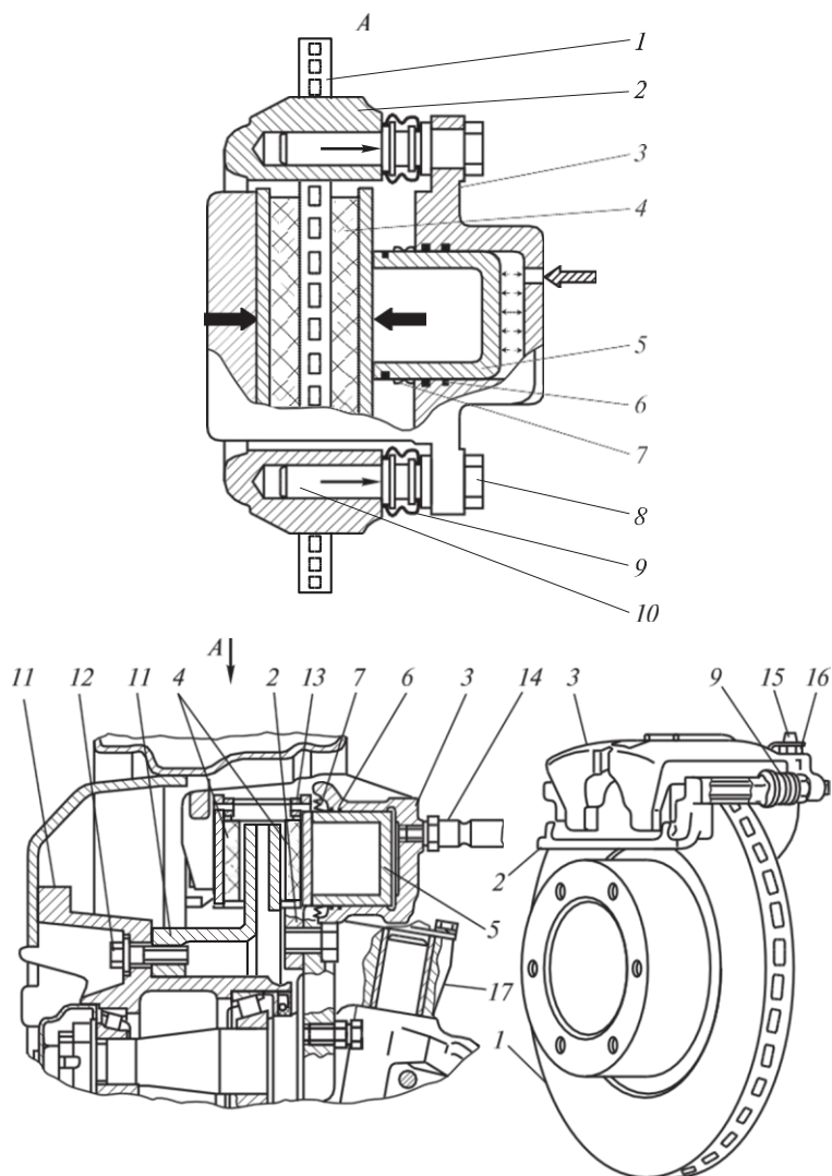
4.78 -сурет. ГАЗ-2752 «Соболь» және ГАЗ-3302 «Газель» автомобильдері алдыңғы дөңгелектерінің тежеуіш тетіктері:
