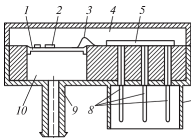
2.67 сур. Ауаның абсолюттік қысымының бергіші:
