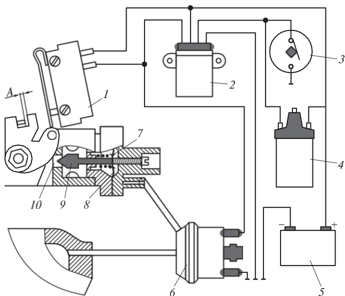
Рис. 2,46, Мәжбүр бос жүрістің экономайзері:
