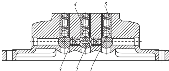
4.21 сур. КамАЗ-141 автомобилі берілісін ауыстыру механизмінің құлыбы мен фиксаторы:
