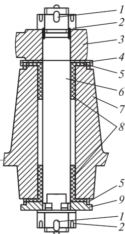
4.61. сурет. ГАЗ-2752 «Соболь» автомобилінің оң жақ маятниктік иіңтірегін орнату:
