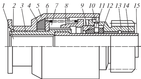
3.11 сур. Байланыстырылмаған жүрістің тіреуіш муфтасы:
