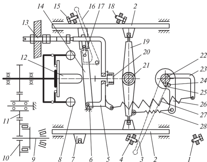
2.79 сур. Ортақ тепкіш реттегіш қондырғысының сызбасы
