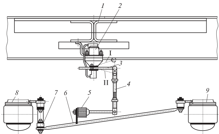
4.91 -сурет. КамАЗ автокөліктерінің тежеуіш күштерін автоматты түрде реттеуішті орнату:
