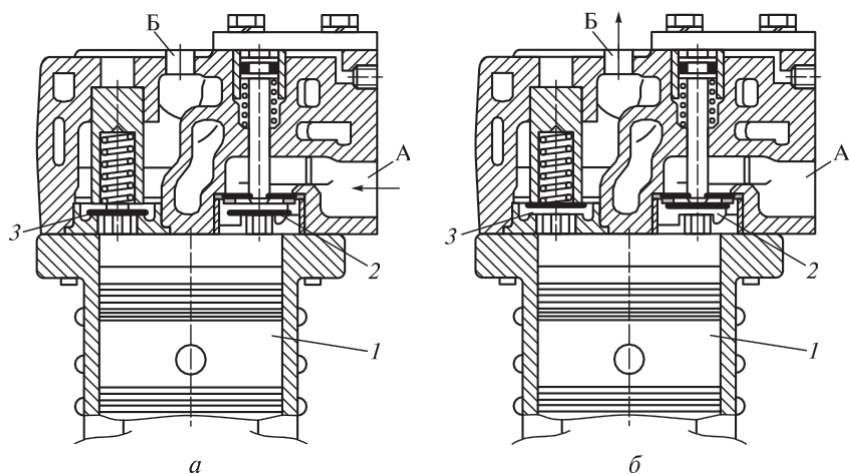
4.95 -сурет. Бірцилиндрлі піспекті біркамералы компрессор жұмысының сызбасы: а — сору тактісі; б — қысу тактісі; 1 — піспек; 2 — кіріс клапаны; 3 — шығыс клапаны; А — кіріс тесігі; Б — шығыс тесігі; —►— ауа ағыны
