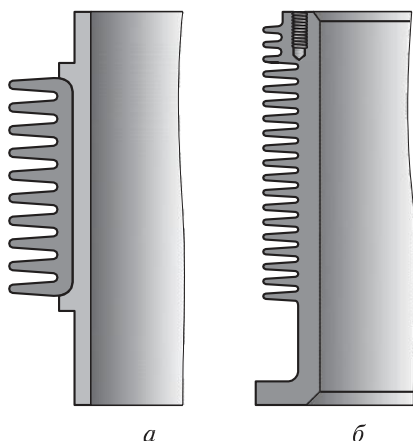
26. сур. Ауа салқындауы бар ІЖҚ қабырғалау түрлері:
