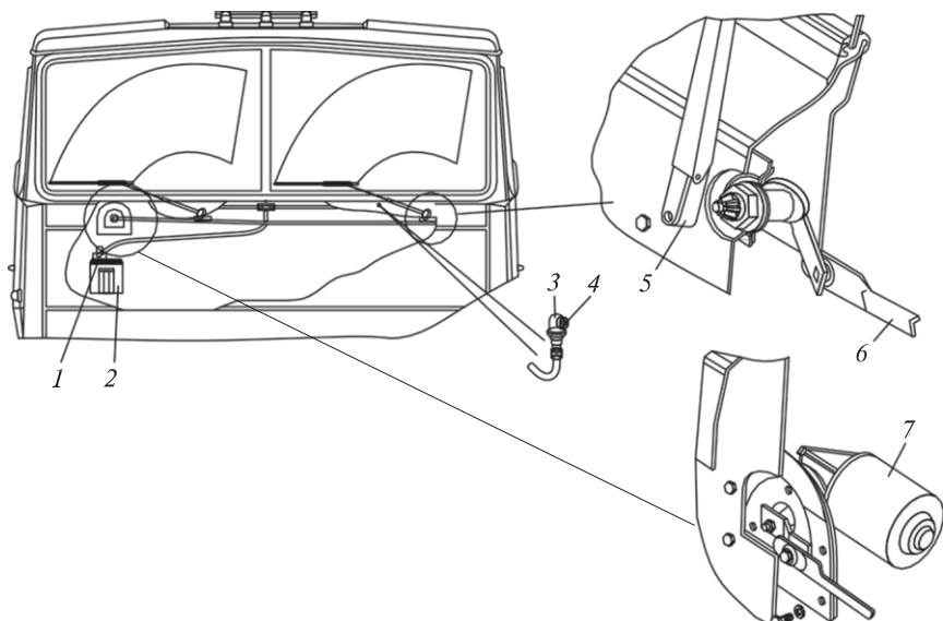
3.14 сур. КамАЗ-5320 жүк көлігінің электр шыны жуғышы:
