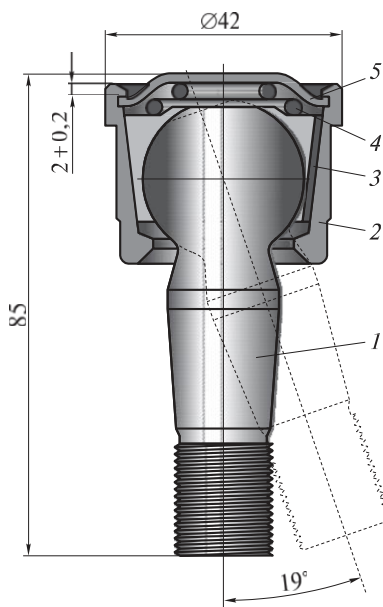
4.62. сурет. ГАЗ-2752 «Соболь» және ГАЗ-3302 «Газель» автомобильдерініңменгерік тартымдарының шарлы топсасы: 1 — шарлы сұққы; 2 — топсаның корпусы; 3 — ішпек; 4 — конустық серіппе; 5 — қақпақ
