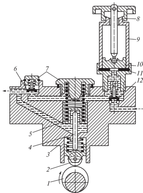
2.74 сур. Төмен қысымды піспектік сорғышы:
