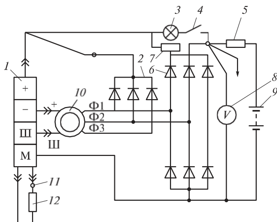
3.38 сур. Генератордың қосылу тізбегіндегі вольтметрді орнату сызбасы: 1 — кернеу реттегіші; 2 — қосымша диодтық белдік; 3 — генераторлық құрылғы жағдайының дабылды шамы; 4 — сөндіргіш; 5 — 30 А сақтандырғышы; 6 — негізгі диодтық белдік; 7, 12 — электр кедергісі; 8 — вольтметр (кернеу көрсеткіші); 9 — аккумулятор батареясы; 10 — генератор; 11 — электролит температурасының қадағасы; Φ1 — Φ3 — фазалар; М, Ш, +, — клеммалар
