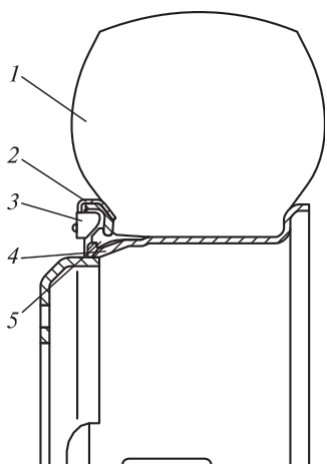
4.125 -сурет. КамАЗ-5320 автомобилінің дөңгелегі: 1 — дөңгелек; 2 — кольцо бортовое; 3 — груз балансирующий; 4 — тоғын, сваренный с дис- ком; 5 — кольцо замочное
