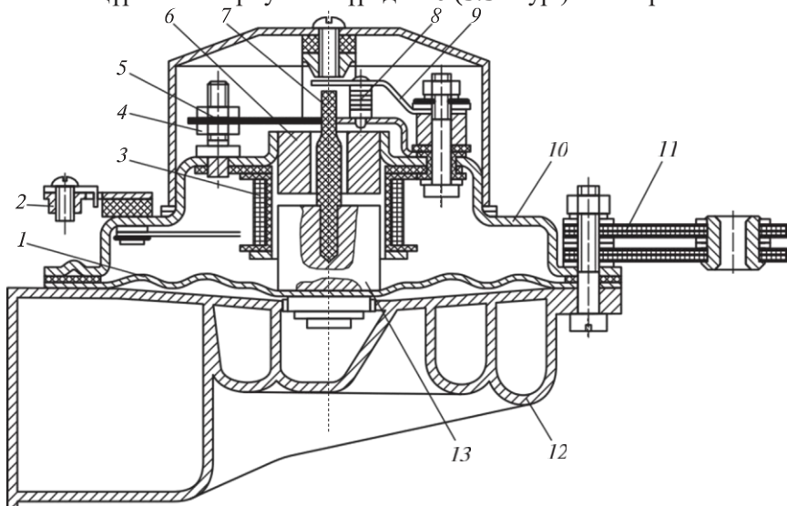
3.31 сур. Үндестік дыбыстық сигнализация:
