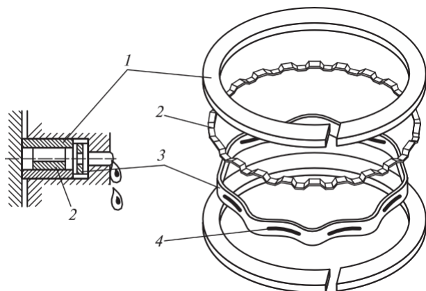
213 сур. Құрама май жинағыш бұдақтар:
