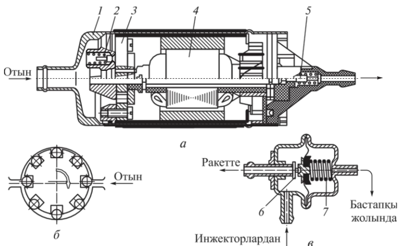
2.59 сур. ЗМЗ-4062.10 доңгелектік типті қозғалтқыштың электрлік бензосорғышы: а — құрылымдық қондырғы; б — сорғыштың айдау торабы жұмысының қағидасы; в — қысымның реттегіші; 1 — корпус; 2 — сақтандырғыш клапан; 3 — сорғыштың доңгелектері; 4 — зәкір; 5 — кері клапан; 6 — тиек клапан; 7 — серіппе; «е» — механизм айналуы
