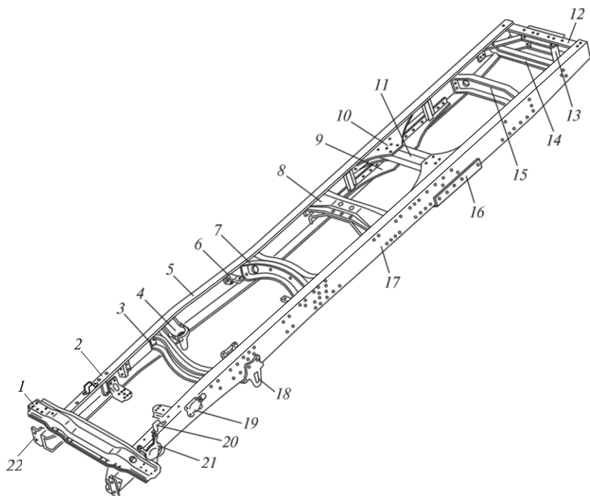
4.112 -сурет. КамАЗ-5320 автомобилінің рамасы:
