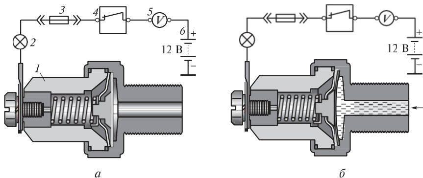
3.37 сур. Май қысымын апатты төмендету қадағасы: а — қосылудың дабылды шамы; 1 — қадаға; 2 — дабылды шам; 3 — сақтандырғыш; 4 — тұтандырудың сөндіргіш; 5 — кернеу көрсеткіші; 6 — аккумулятор батареясы; б — сөндірудің дабылды шамы: —» — май қысымы
