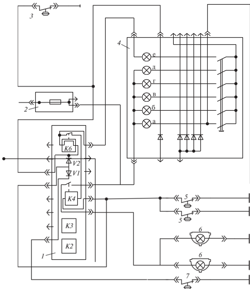
3.27 сур. Тежегіштің жарық дабылын қосу сызбасы:
