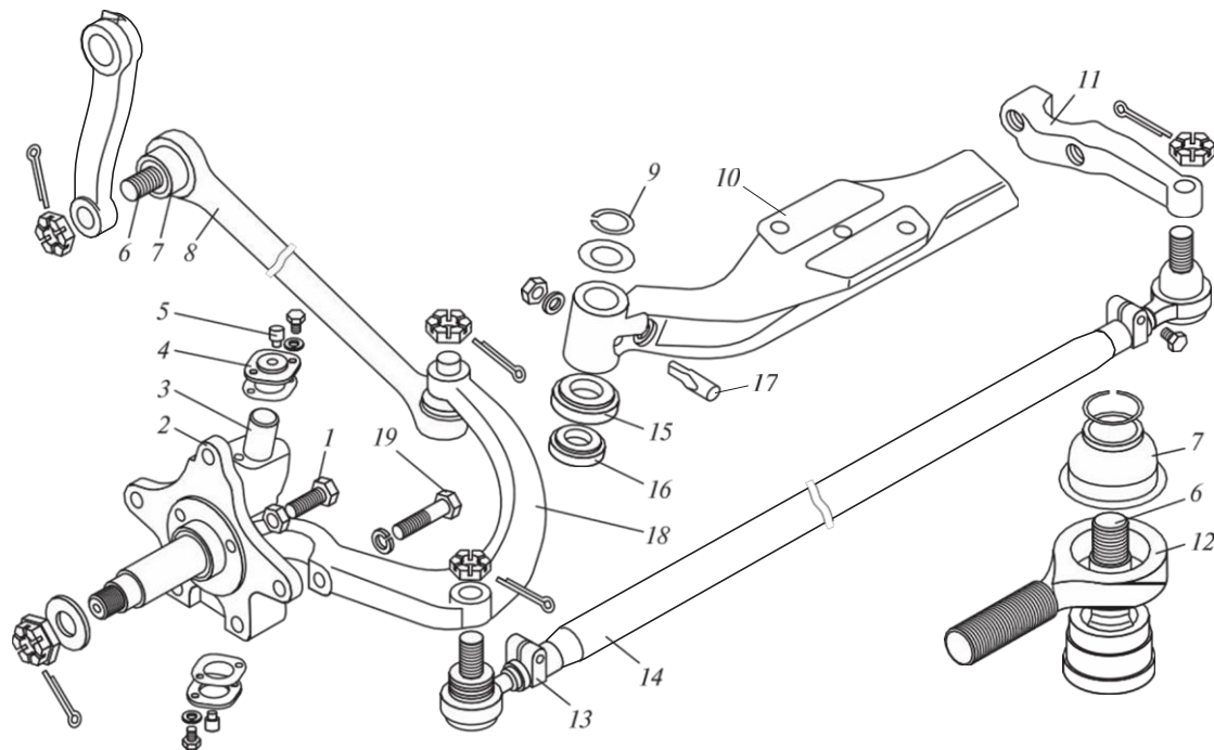
4.63. сурет. ГАЗ-3302 «Газель» автомобилінің меңгерік жетегі:
