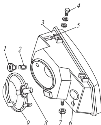
3.18 сур. ЗИЛ-5301 автомобилінің тік бұрышты пішінді фарасы:
