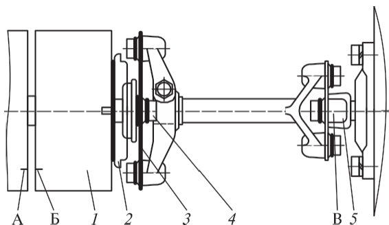
2.80 сур. Отынды бүрку алдын алуғағы автоматты жалғастырғыштың жетегі: 1 — бүрку алдын алуғағы автоматты жалғастырғышы; 2 — жетектің жетелейтін жартылай жалғастырғышы; 3 — жетектің жетелейтін жартылай жалғастырғышының алдыңғы фланеці; 4 — бұрандама; 5 — жетектің жетекші жартылай жалғастырғышының артқы фланеці; А, Б, В — жоғары қысымды отын сорғышының корпусындағы таңбалар, бүркуді алдын алу жалғастырғышы және жетекші жартылай жалғастырғышының артқы фланеці сәйкесінше
