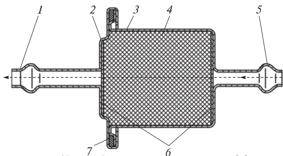
2.60 сур. Отынды ақтап тазарту сүзгісі:
