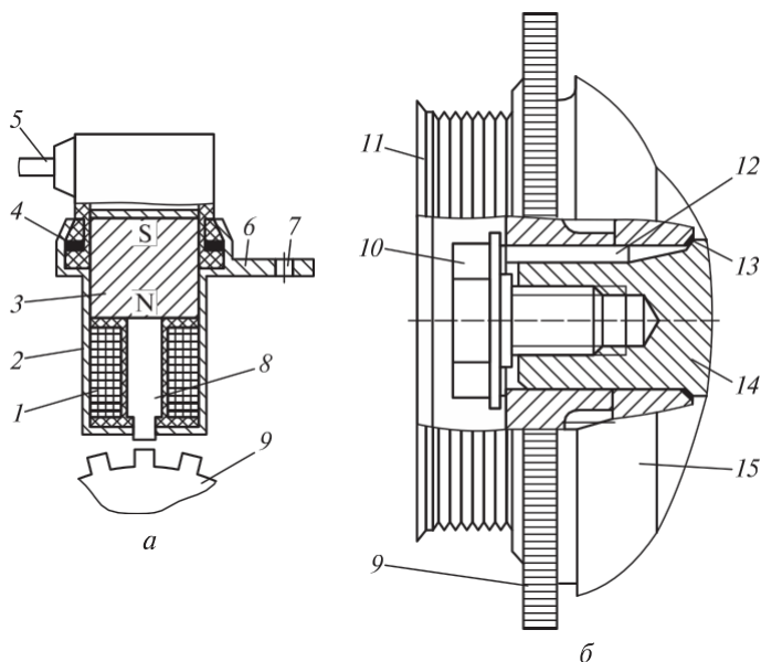
Рис. 2.70. Датчик частоты вращения коленчатого вала: а — размещение датчика; б — зубчатый венец; 1 — обмотка катушки; 2 — корпус; 3 — постоянный магнит; 4 — уплотнитель; 5 — провод; 6 — кронштейн крепления; 7 — отверстие крепления; 8 — магнитный сердечник; 9 — диск синхронизации; 10 — стяжной болт; 11 — шкив-демпфер; 12 — шпонка; 13 — резиновое кольцо; 14 — коленчатый вал двигателя; 15 — маховик
