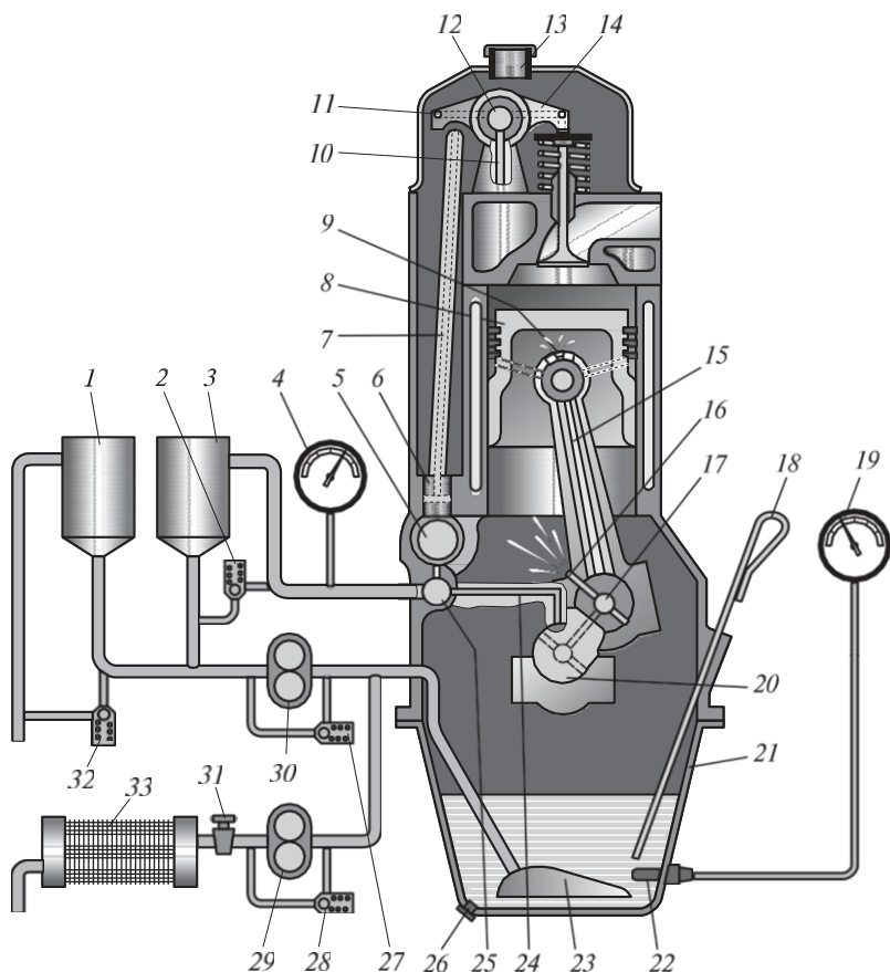
2.32 сур. Майлау жүйесінің құрылғысы:
