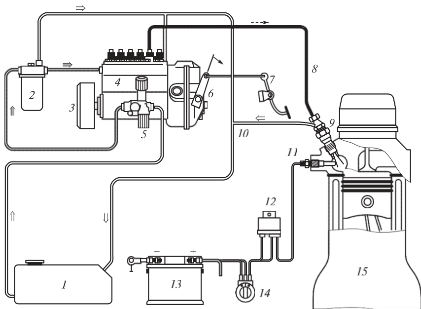
2.72 сур. Дизельдің отын беру жүйесі:
