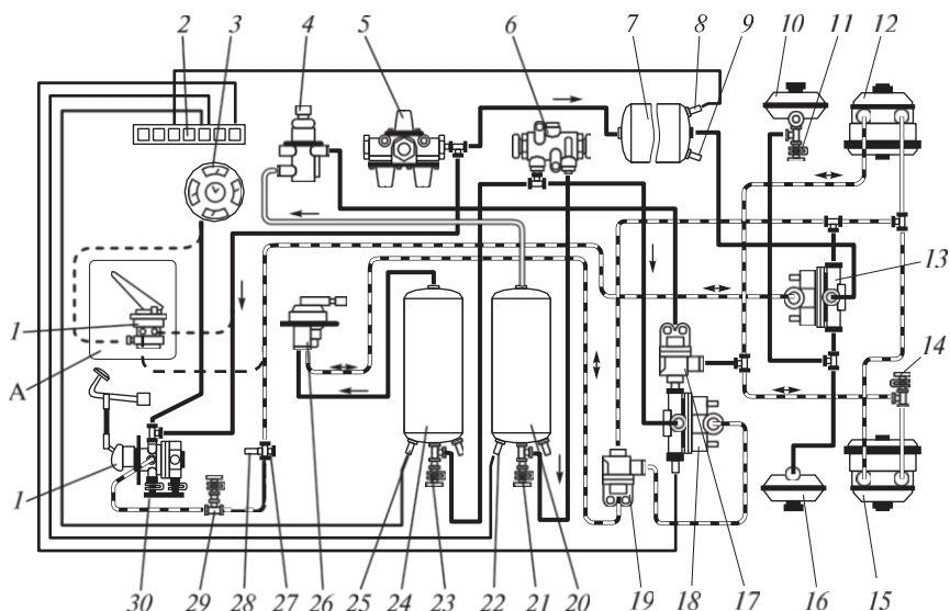
4.104 -сурет. Артқы арба жұмыс жеңеуіші жетегі контурының сызбасы: 1 — екі секциялы тежегіш қран; 2 — бақылау шамдары блогі; 3 — КР-129 құрамдастырылған аспабы; 4 — апаттық тежеу шүмегі; 5 — үш қорғағышты клапан; 6 — қосарланған қорғағышты клапан; 7 — артқы арба жұмыс жеңеуіштері жетегі контурының баллоны (ресивер); 8, 22, 25 — қысымның апаттық төмендеуінің бергіші; 9 — конденсат ағызу клапаны; 10, 16 — тежеу камералары; 11, 14, 21, 23, 29, 30 — шығысты бақылау клапандары; 12, 15 — қуат аккумуляторлы тежеуіш камералар; 13, 18 — тездеткіш клапандар; 17, 19 — екімагистральді клапандар; 20 — апаттық тежеу контуры баллоны; 24 — тұруға арналған тежеуіш контурының баллоны; 26 — тұруға арналған тежеуіш шүмегі; 27, 28 — қысым датчиктері; А — екісекциялы тежеуіш шүмегінің нұсқасы
