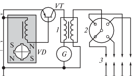
2.91 сур. Магнитэлектрлік бергішті қолдана отырып бастапқы тізбектің үзілуінің түйіспесіз жүйесінің сызбасы:
